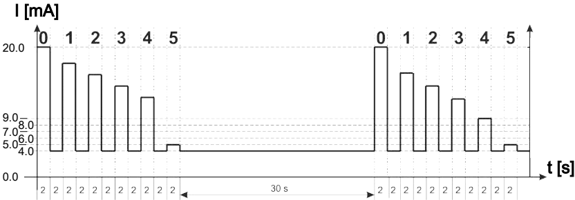
Fig. 28: Example: HDA.ISO analogue output
