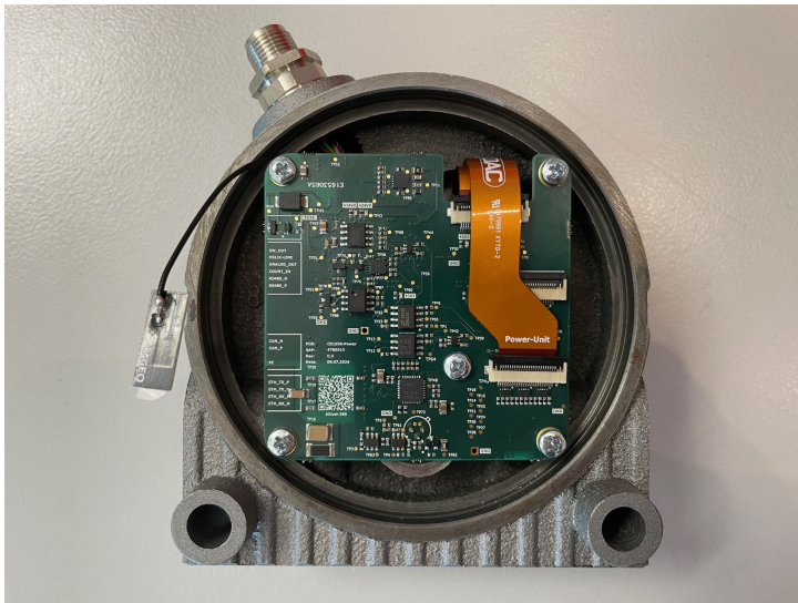
CS1500 Rückansicht
