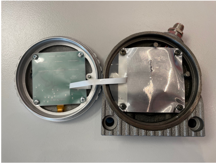
CS1500 Frontansicht
