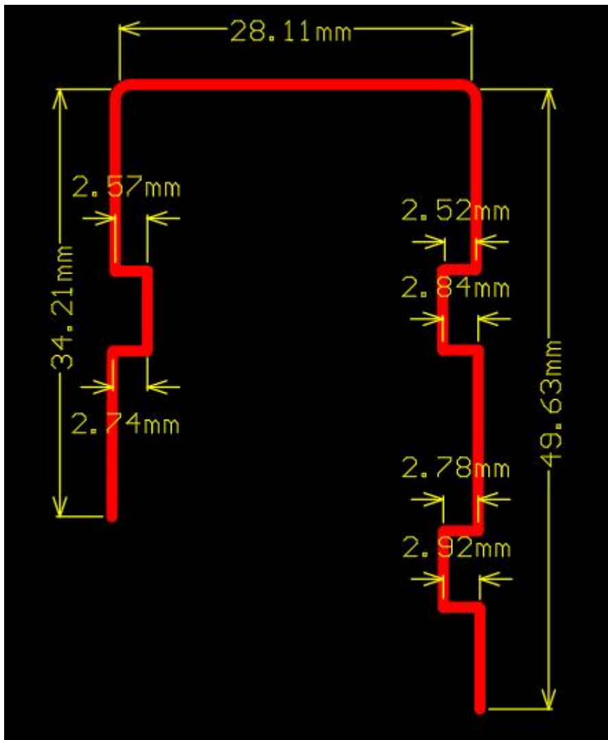
Antenna size(mm)
