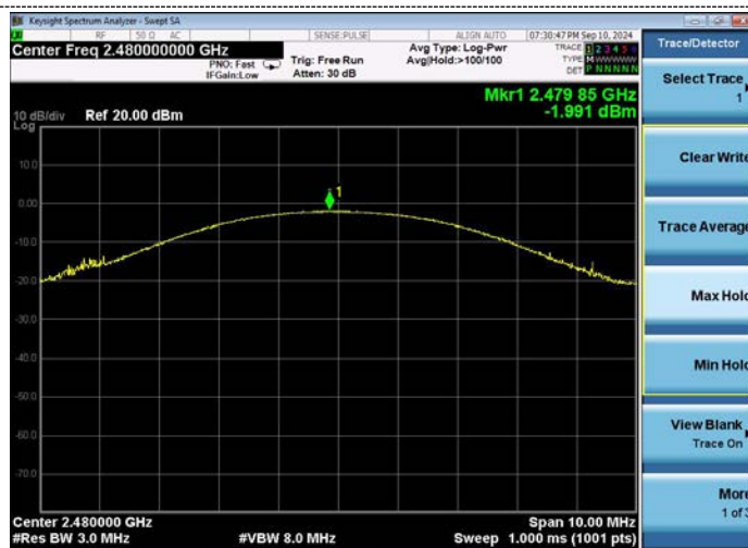
GFSK(CH78)
