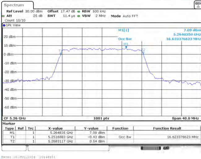
11A-Ant1-5260
