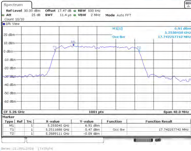
11AC20MIMO-Ant1-5260
