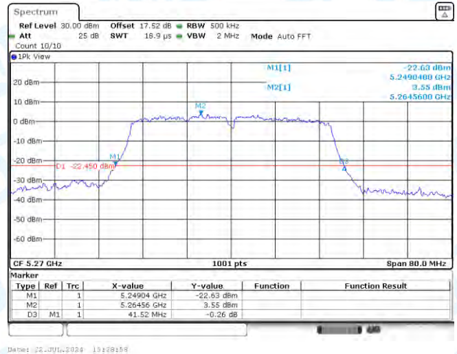
11N40MIMO-Ant2-5270
