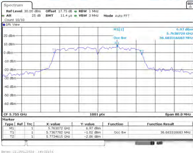
11N40MIMO-Ant1-5755
