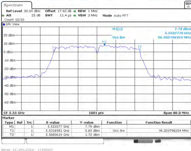
11N40MIMO-Ant1-5550
