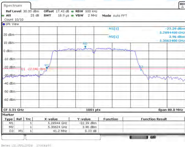
11N40MIMO-Ant1-5310
