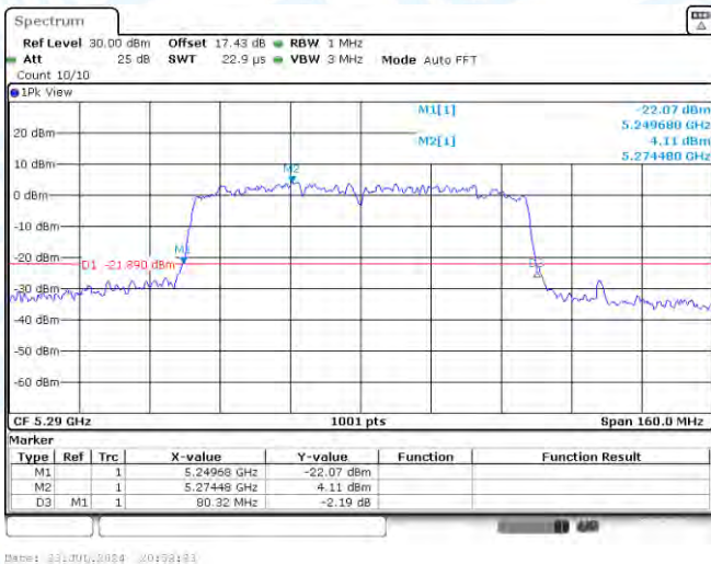
11AC80MIMO-Ant1-5290
