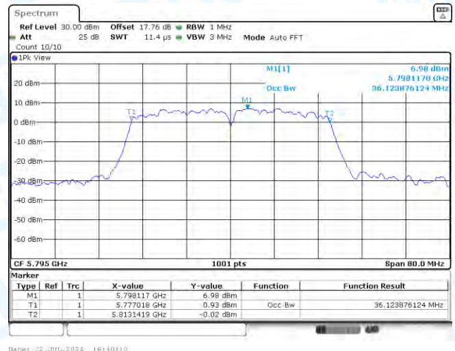
11N40MIMO-Ant2-5795
