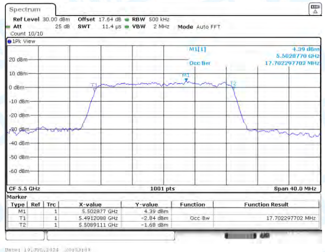
11N20MIMO-Ant2-5500
