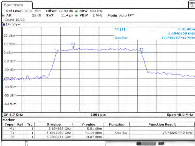
11N20MIMO-Ant1-5700
