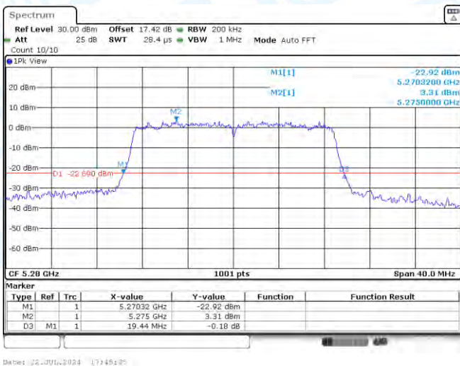
11AC20MIMO-Ant1-5280
