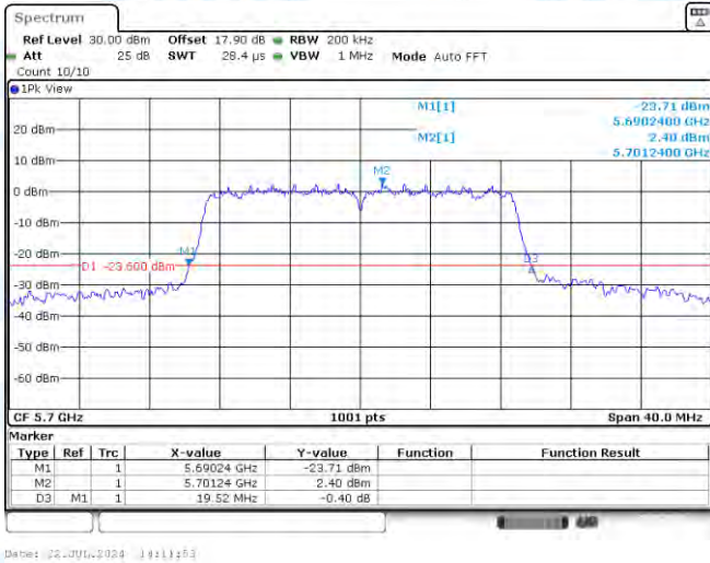
11N20MIMO-Ant1-5700
