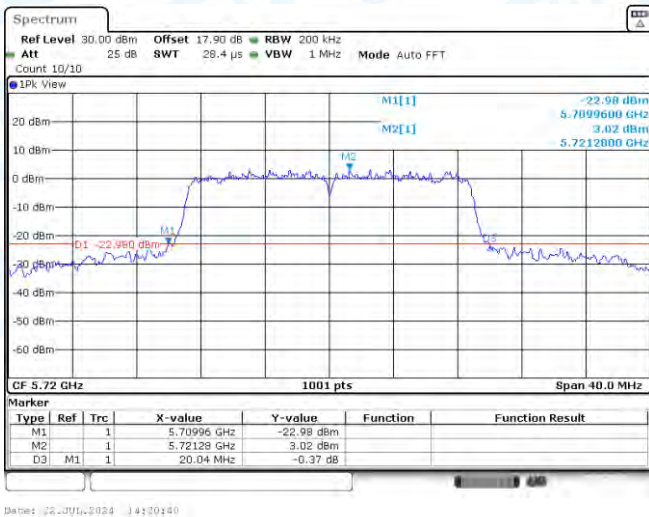
11N20MIMO-Ant1-5720
