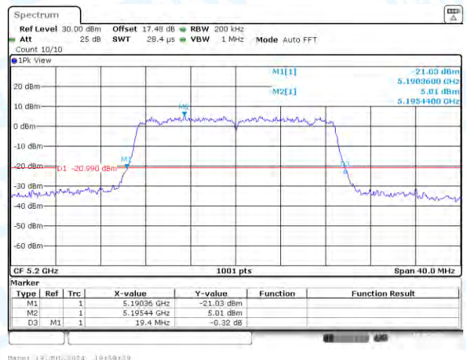
11N20MIMO-Ant2-5200
