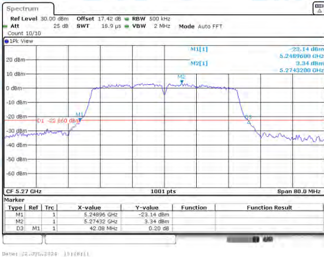
11N40MIMO-Ant1-5270
