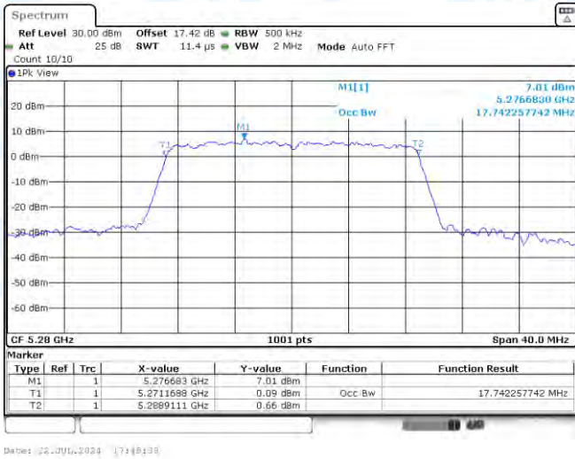
11AC20MIMO-Ant1-5280
