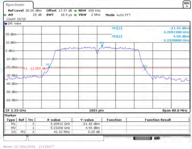
11N40MIMO-Ant2-5230
