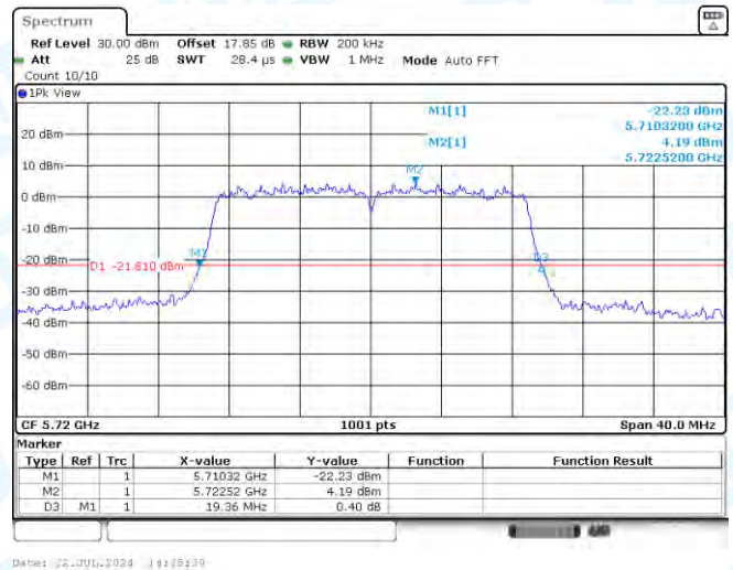
11N20MIMO-Ant2-5720
