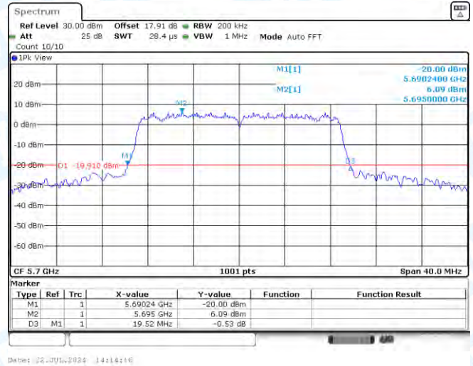
11N20MIMO-Ant2-5700
