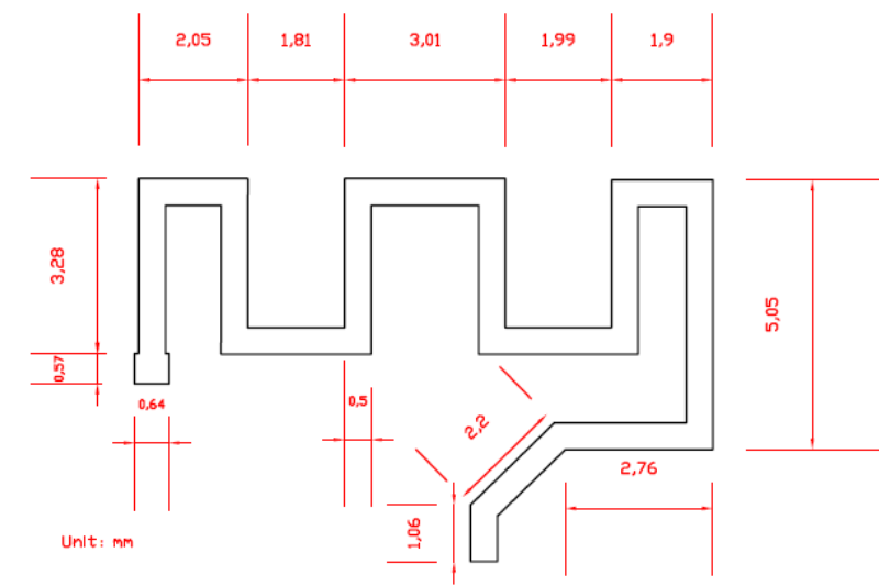
图 1 尺寸图 Figure 1 Size diagram
