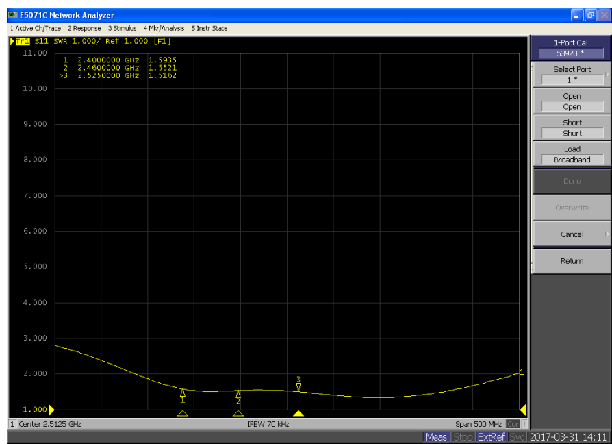
图 3 驻波比测试图 FIG. 3 VSWR test diagram
