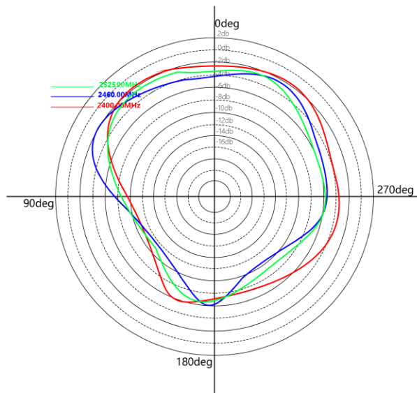
图 5 XOZ 平面天线增益图 Figure 5. Gain of xOZ plane antenna
