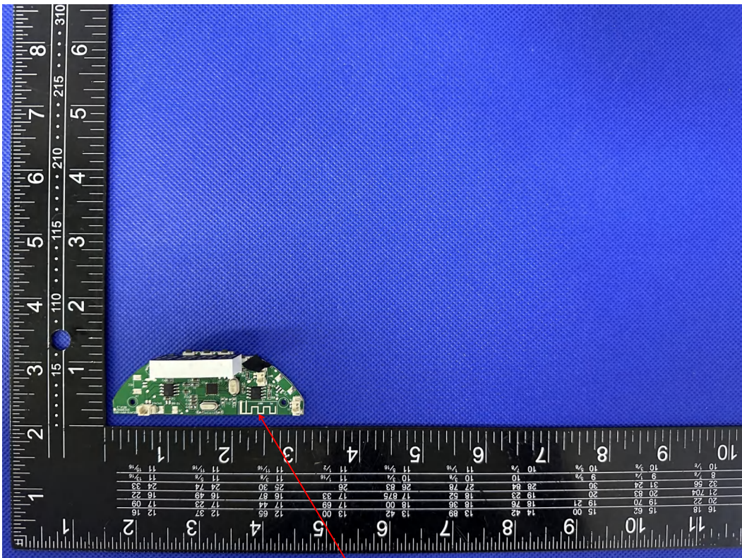
BT ANT
