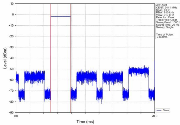
GFSK_DH5_HOPP_Ant1_NTNV
