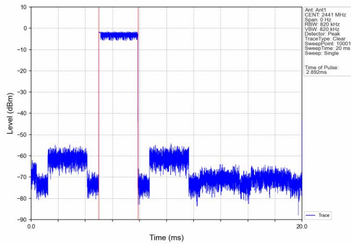
8DPSK_3DH5_HOPP_Ant1_NTNV
