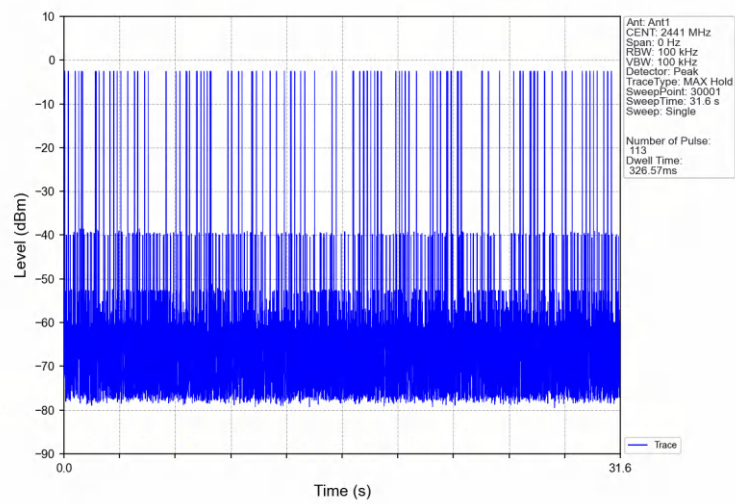
GFSK_DH5_HOPP_Ant1_NTNV
