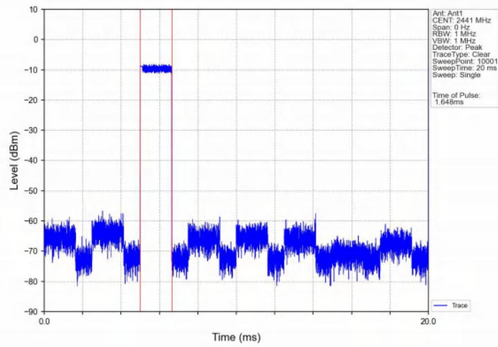
8DPSK_3DH3_HOPP_Ant1_NTNV
