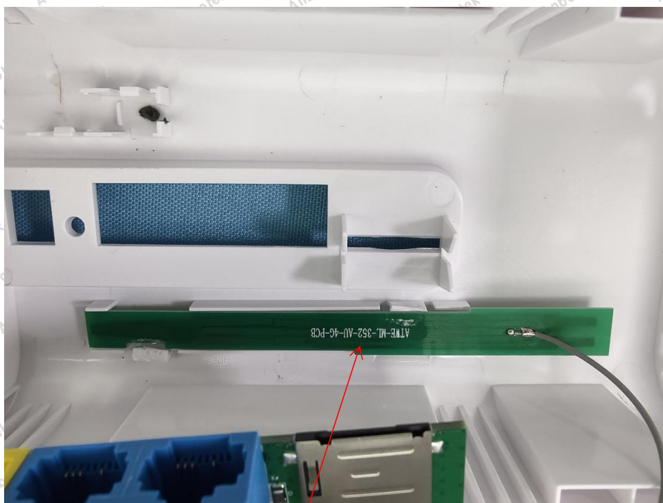
LTE-DIV-ANT
