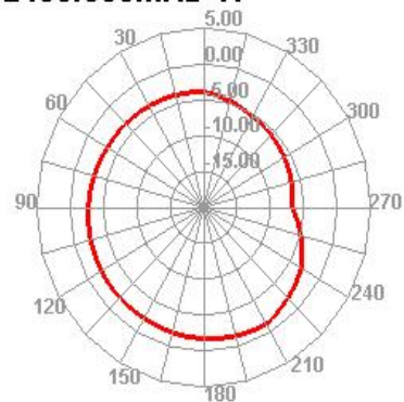
2400.000MHz H
