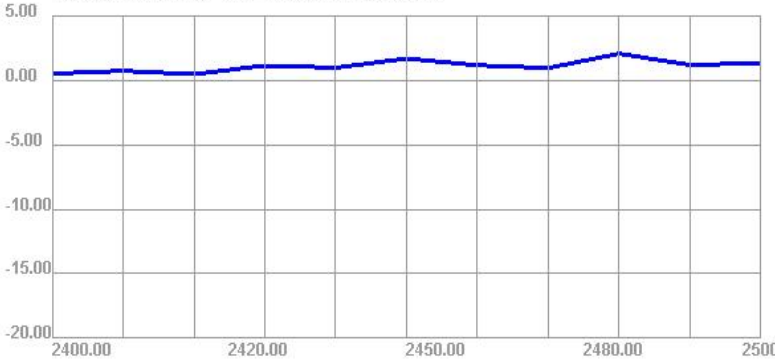
2400.00MHz - 2500.00MHz Efficiency
