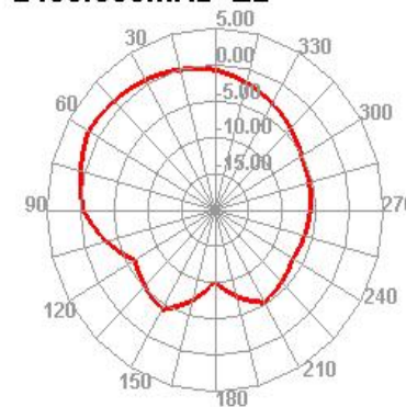
2450.000MHz E2
