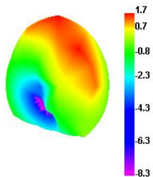
2450.000MHz
