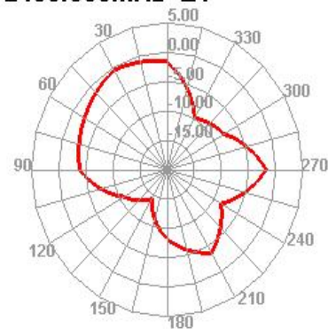
2400.000MHz E1
