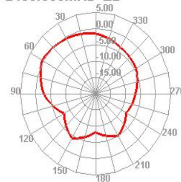
2400.000MHz E2
