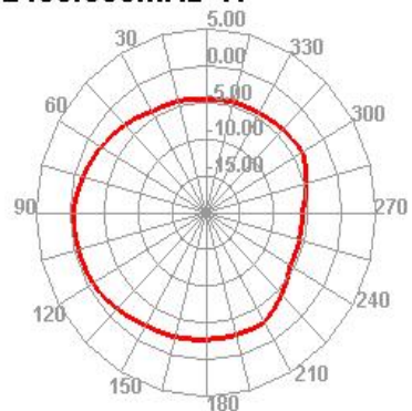
2450.000MHz H
