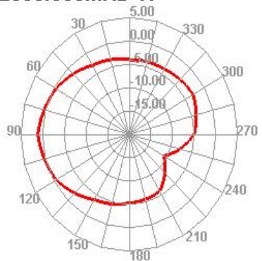
2500.000MHz H
