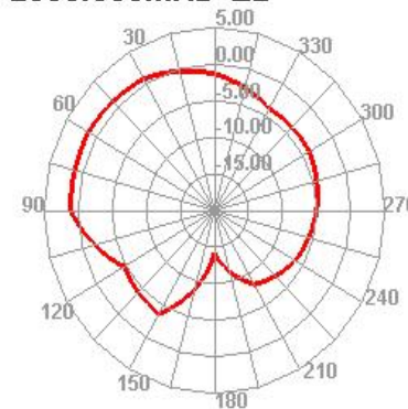
2500.000MHz E2
