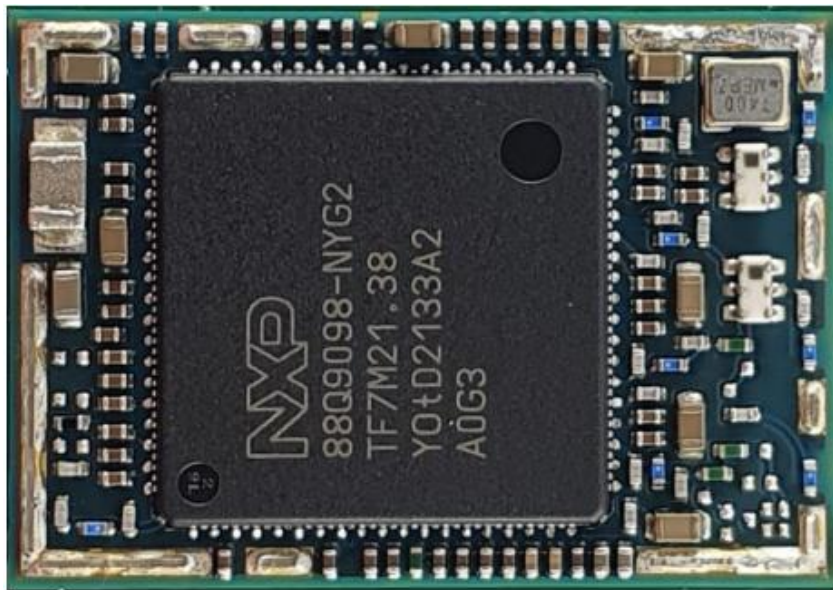
Abbildung 17: ublox module internals
