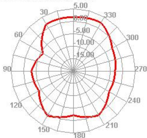
5500.000MHz E2
