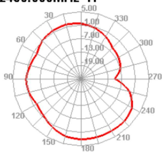
2450.000MHz H
