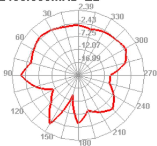
2450.000MHz E2
