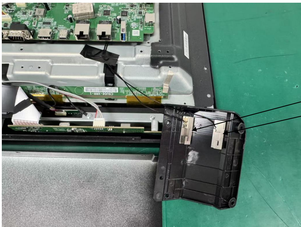
NXP8997 ANT
