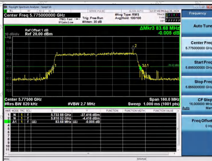
11AC80SISO-Ant1-5775
