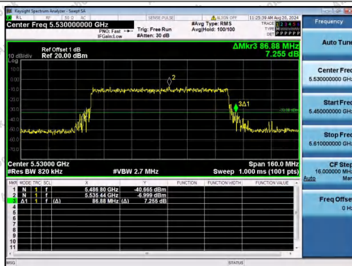
11AC80SISO-Ant1-5530
