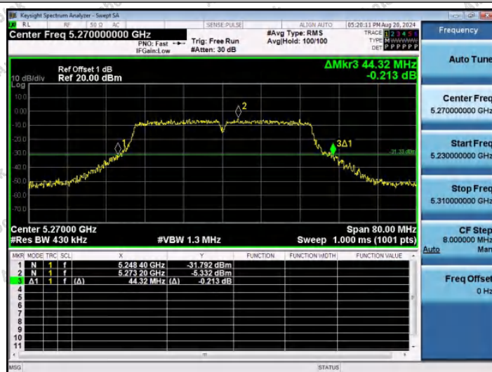
11N40SISO-Ant1-5270
