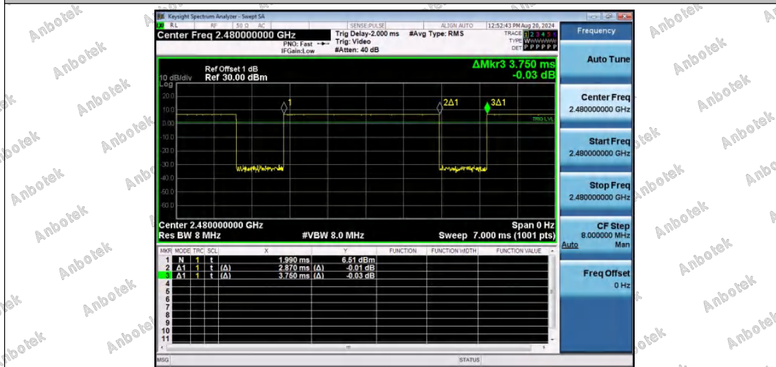
NTNV-DH5-Ant1-2480
