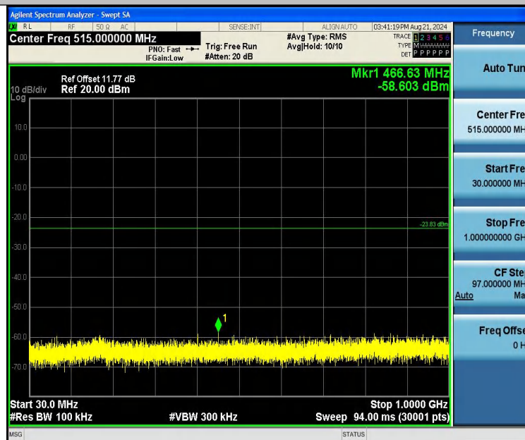
BLE_2M-Ant1-2440-30~1000-PASS
