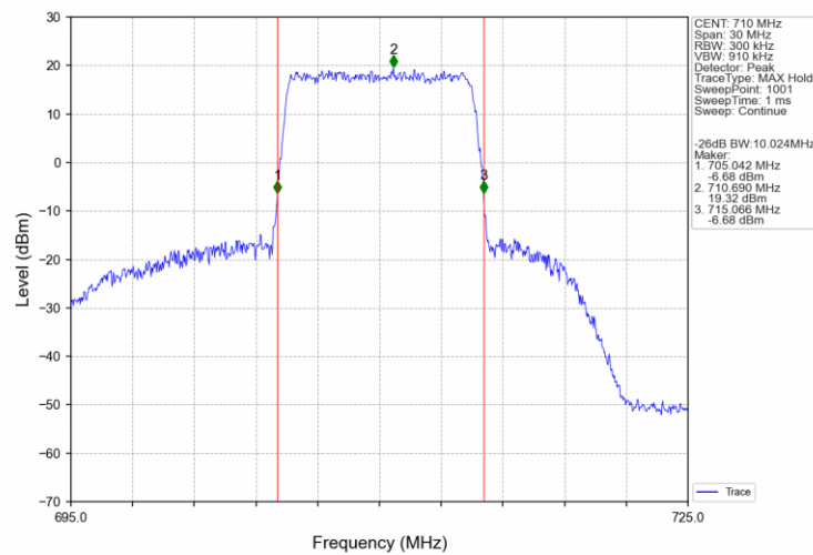
Band17 10MHz QPSK MCH 710MHz RB 50 0 NTV
