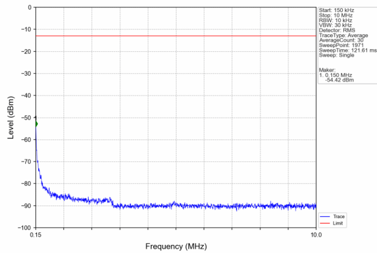
Band5_3MHz_QPSK_HCH_847.5MHz_RB_1_0_NTNV
