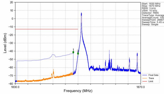
Band2_20MHz_QPSK_LCH_1860MHz_RB_1_0_NTNV
