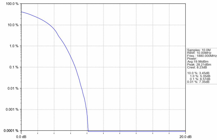
Band2_20MHz_16QAM_MCH_1880MHz_RB_100_0_NTNV
