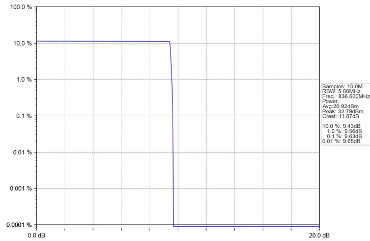
GSM850_GSM_MCH_836.6MHz_GSM_NTNV
