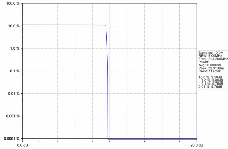
GSM850_GSM_LCH_824.2MHz_GSM_NTNV
