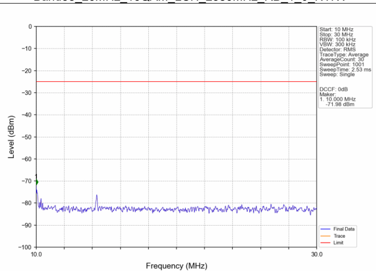
Band38_20MHz_16QAM_LCH_2580MHz_RB_1_0_NTNV
