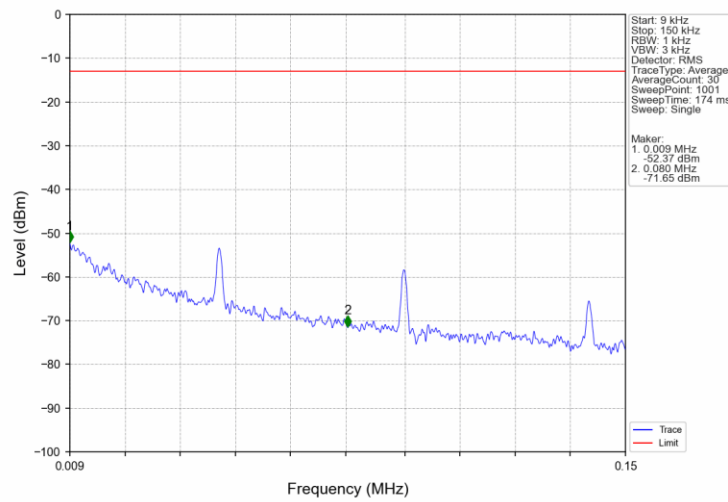
Band2_20MHz_16QAM_HCH_1900MHz_RB_1_0_NTNV
