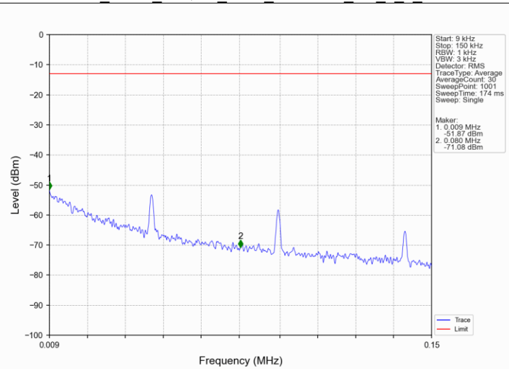
Band2_3MHz_16QAM_MCH_1880MHz_RB_1_0_NTNV
