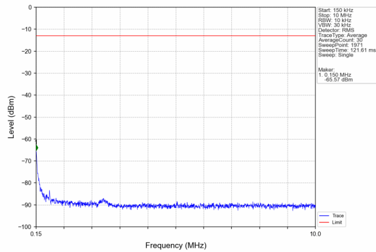
Band2_3MHz_QPSK_HCH_1908.5MHz_RB_1_0_NTNV
