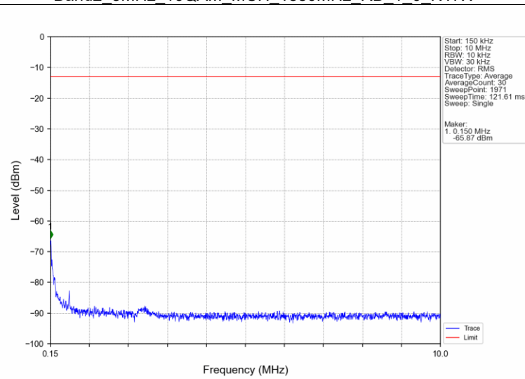
Band2_3MHz_16QAM_MCH_1880MHz_RB_1_0_NTNV
