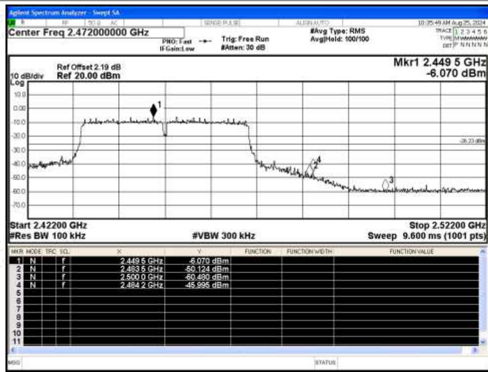
Band Edge NVNT n40 2452MHz Ant Emission
