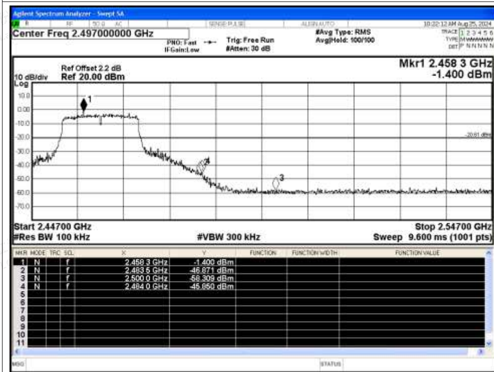
Band Edge NVNT g 2462MHz Ant Emission
