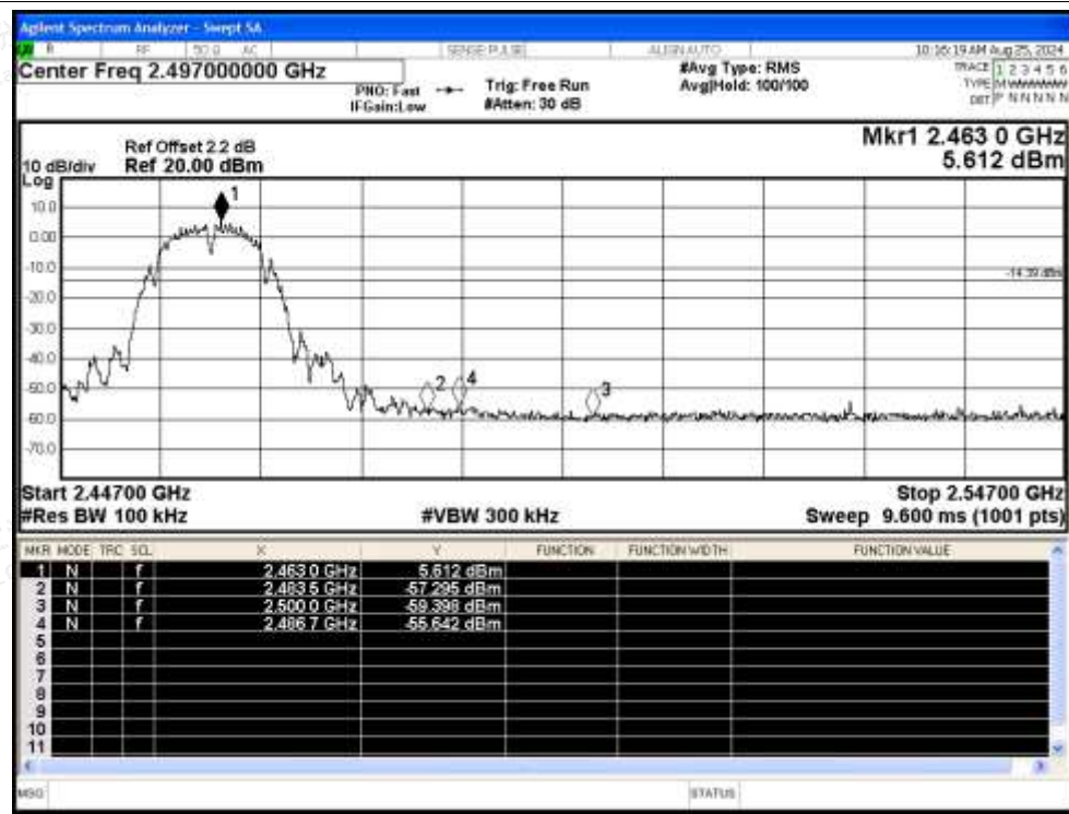
Band Edge NVNT b 2462MHz Ant Emission
