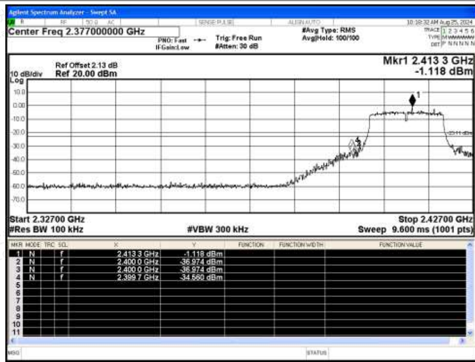
Band Edge NVNT g 2412MHz Ant Emission
