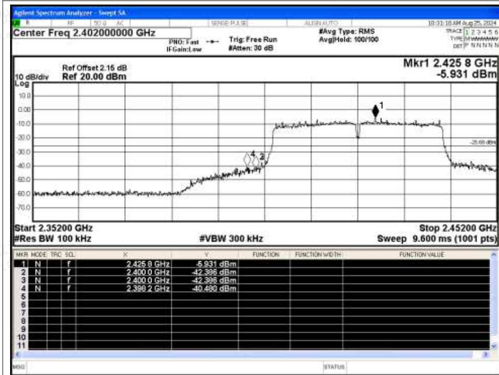
Band Edge NVNT n40 2422MHz Ant Emission
