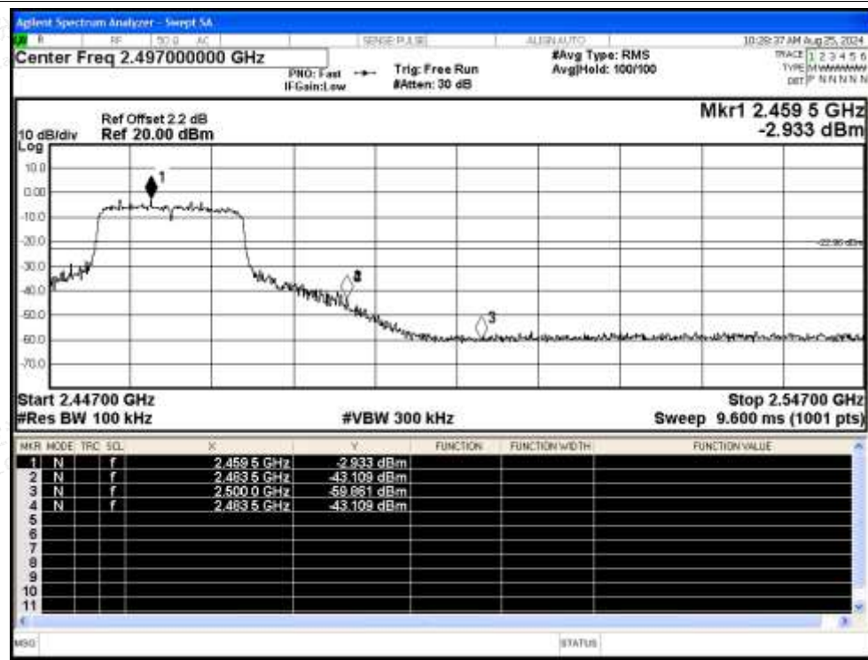
Band Edge NVNT n20 2462MHz Ant Emission
