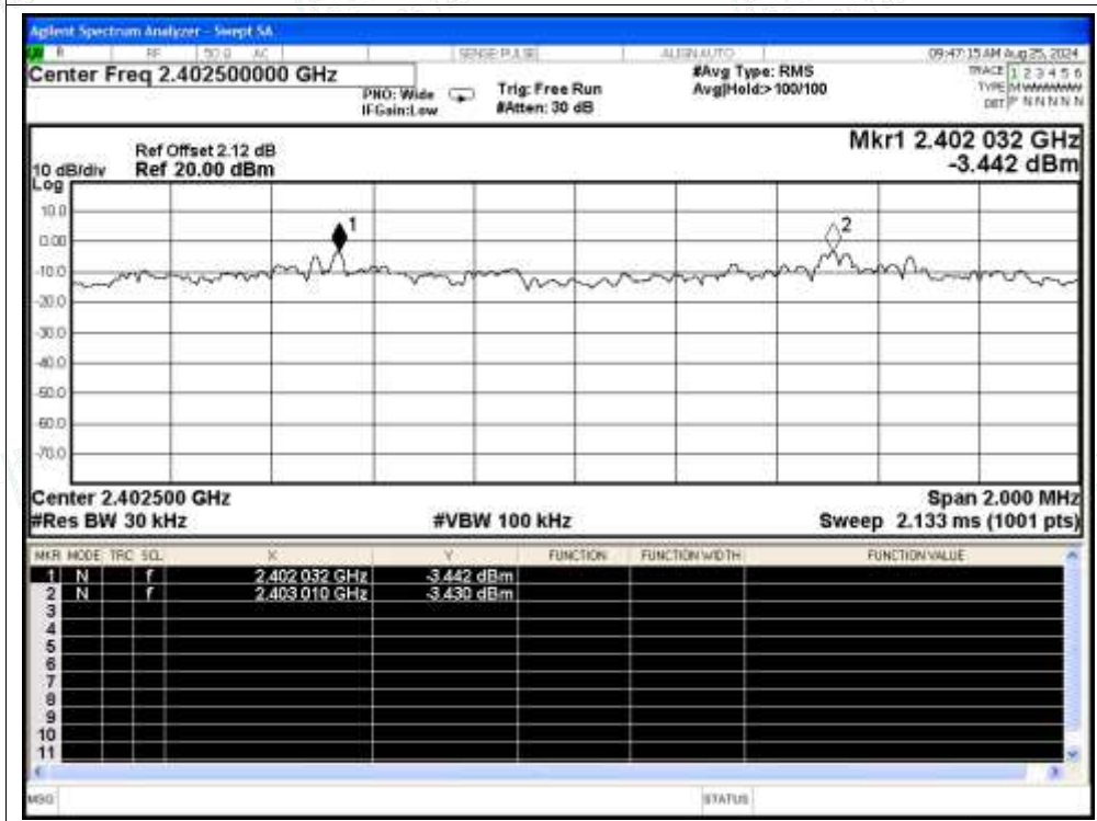
CFS NVNT 3-DH5 2402MHz Ant
