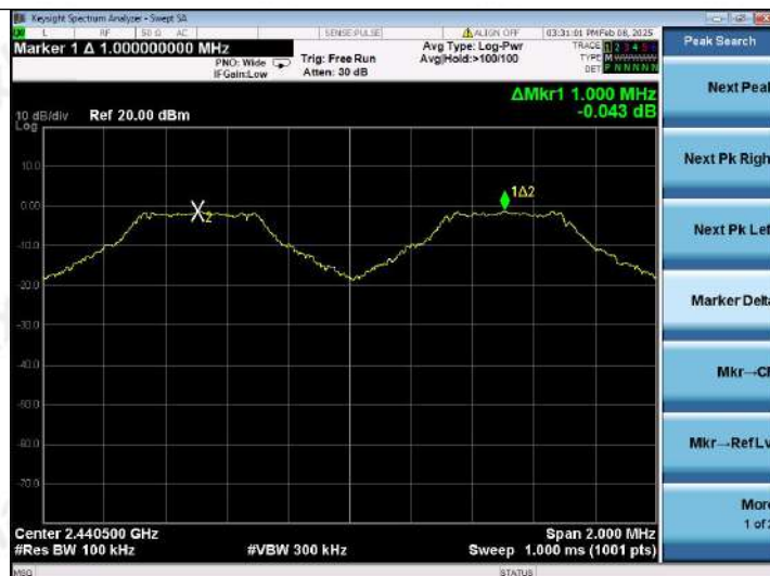
GFSK
