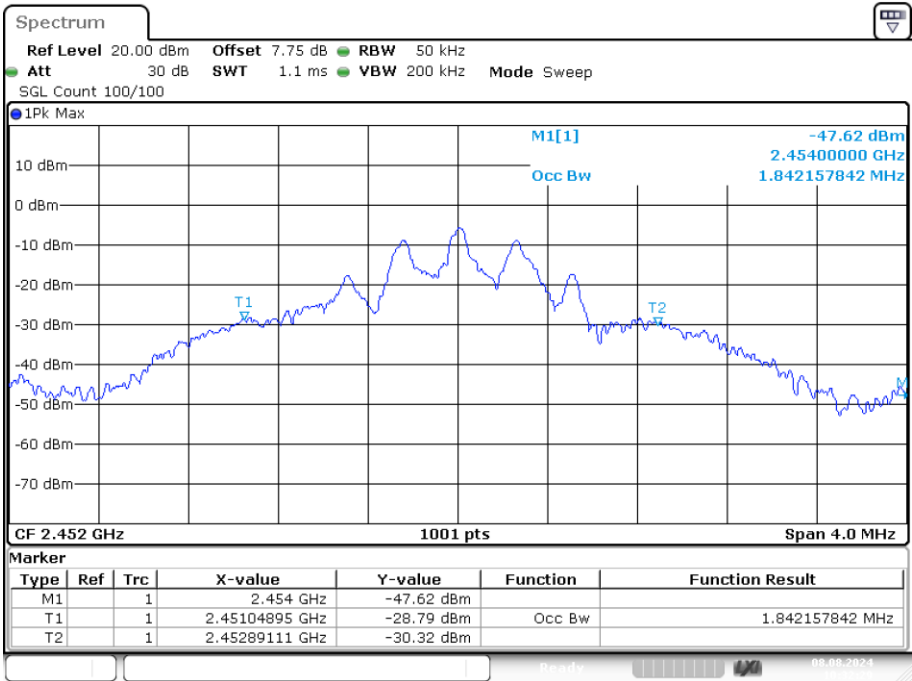
OBW NVNT GFSK 2452MHz Ant1
