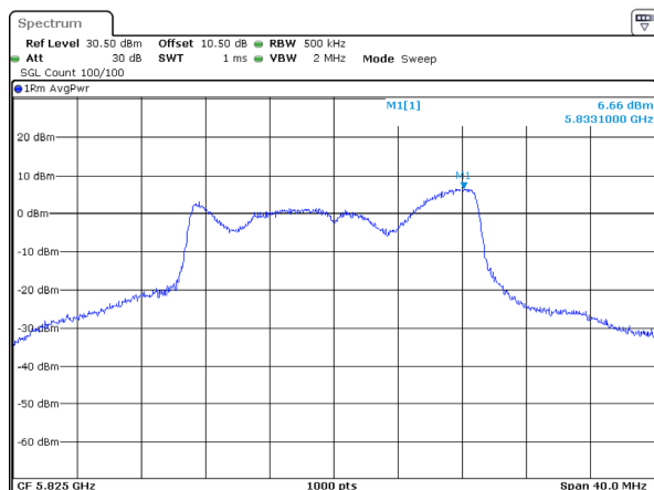
802.11ac20_5825MHz_Chain 2
