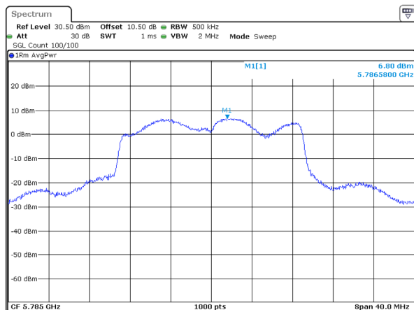
802.11ac20_5785MHz_Chain 3
