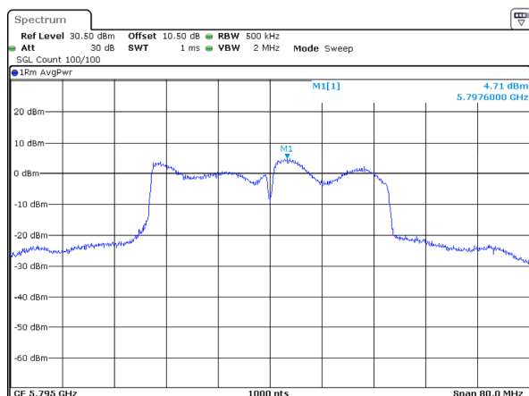
802.11ac40_5795MHz_Chain 2
