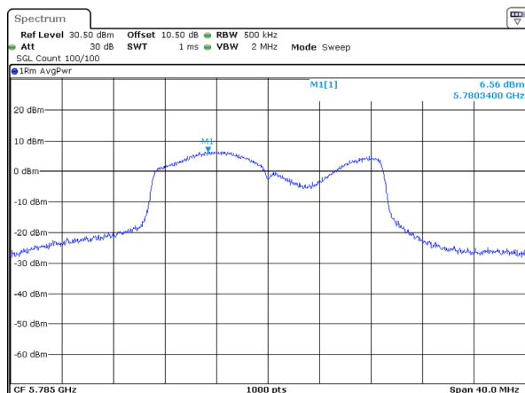
802.11ac20_5785MHz_Chain 2
