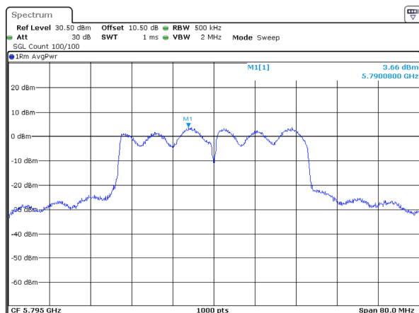
802.11ac40_5795MHz_Chain 3
