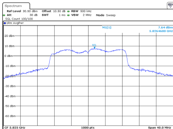
802.11ac20_5825MHz_Chain 3
