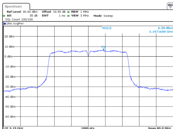
802.11ac40_5190MHz_Chain 3
