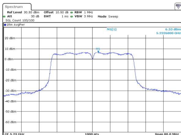
802.11ac40_5230MHz_Chain 3
