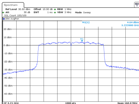
802.11ac80_5210MHz_Chain 3
