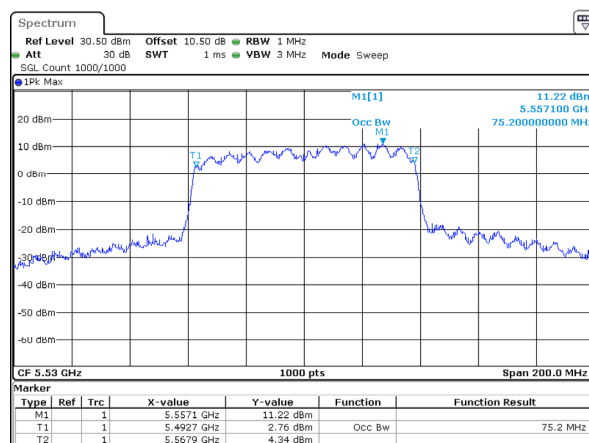
802.11ac80_5530MHz_Chain 3
