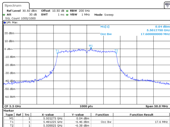
802.11ac20_5500MHz_Chain 0
