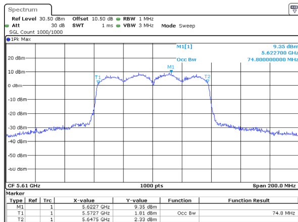
802.11ac80_5610MHz_Chain 1
