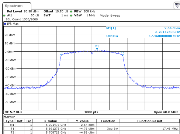
802.11ac20_5700MHz_Chain 1
