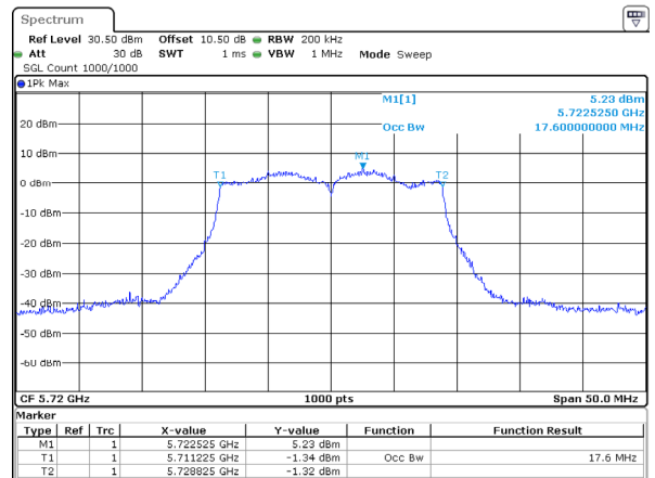
802.11ac20_5720MHz_Chain 3
