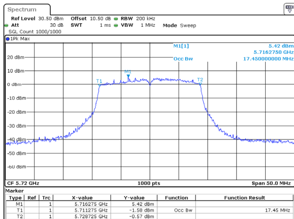
802.11ac20_5720MHz_Chain 1
