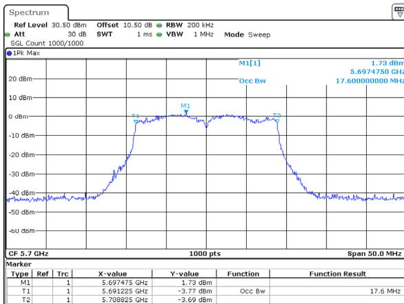
802.11ac20_5700MHz_Chain 3
