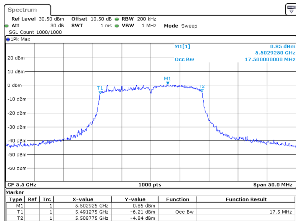
802.11ac20_5500MHz_Chain 1
