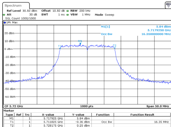
802.11a_5720MHz_Chain 3
