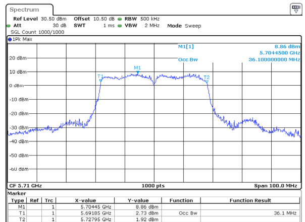
802.11ac40_5710MHz_Chain 0
