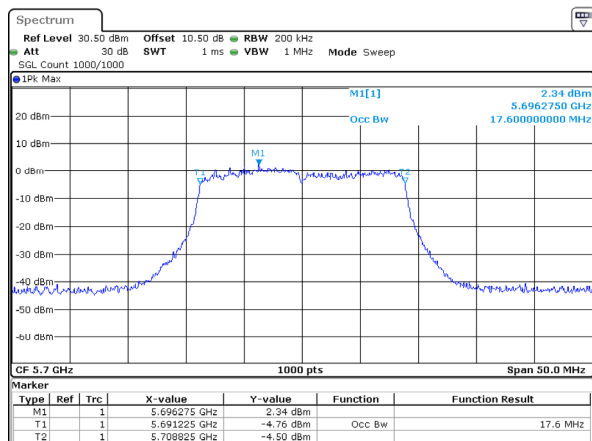
802.11ac20_5700MHz_Chain 0
