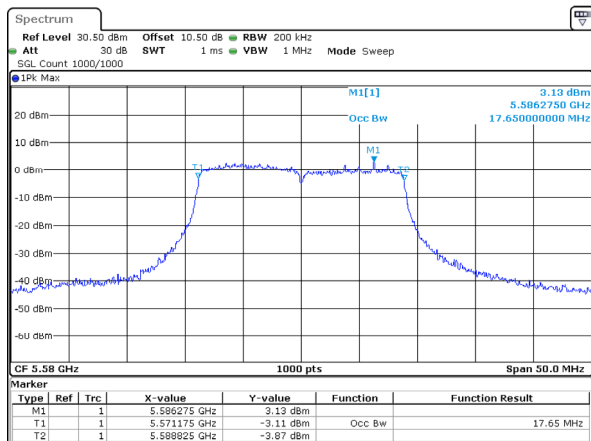
802.11ac20_5580MHz_Chain 1
