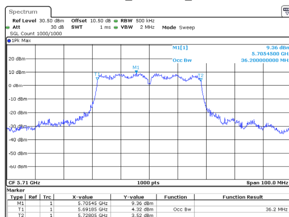
802.11ac40_5710MHz_Chain 3
