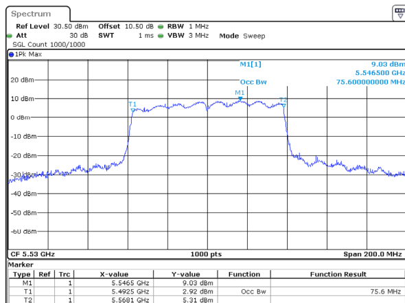
802.11ac80_5530MHz_Chain 0
