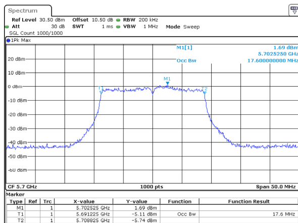
802.11ac20_5700MHz_Chain 2
