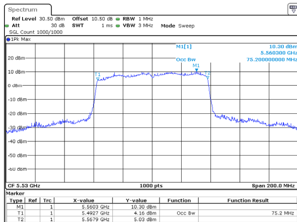
802.11ac80_5530MHz_Chain 1
