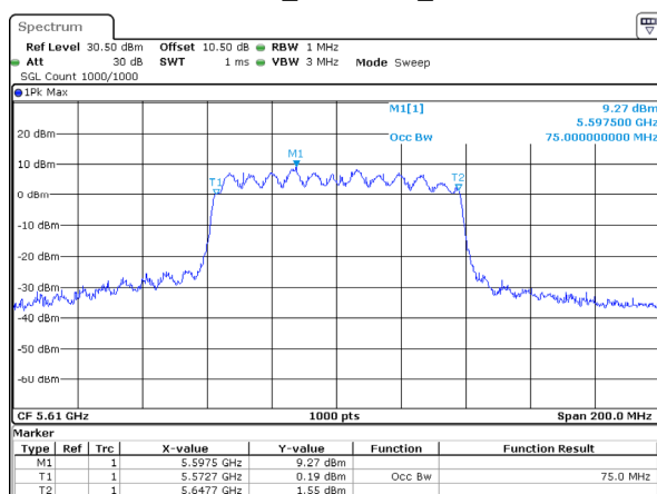
802.11ac80_5610MHz_Chain 3
