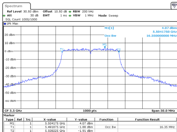
802.11a_5500MHz_Chain 3
