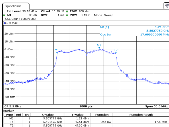
802.11ac20_5500MHz_Chain 3
