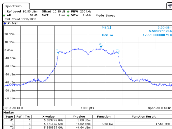
802.11ac20_5580MHz_Chain 3
