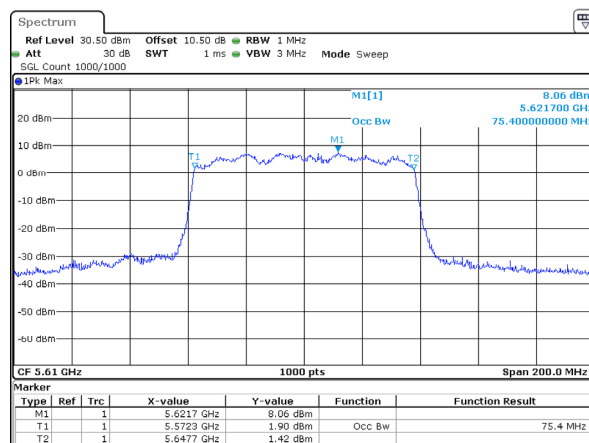
802.11ac80_5610MHz_Chain 2
