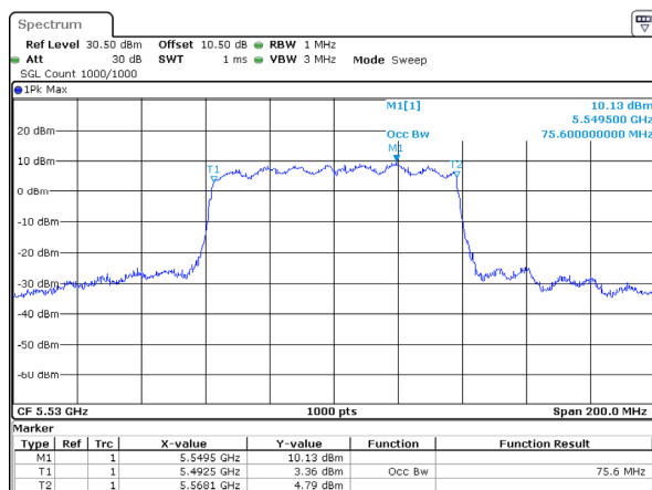
802.11ac80_5530MHz_Chain 2
