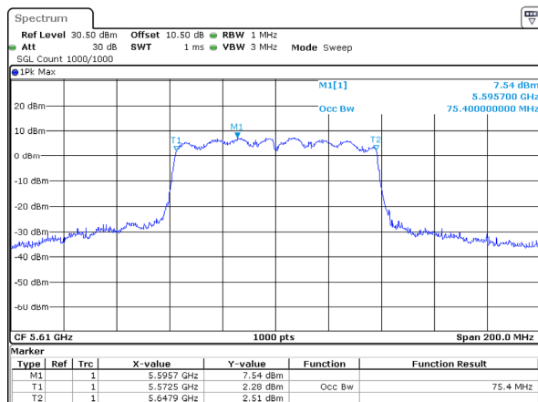
802.11ac80_5610MHz_Chain 0
