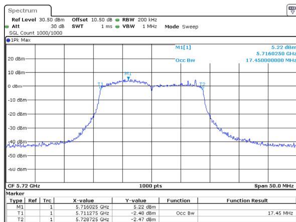
802.11ac20_5720MHz_Chain 2
