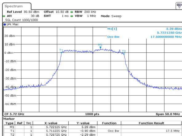
802.11ac20_5720MHz_Chain 0
