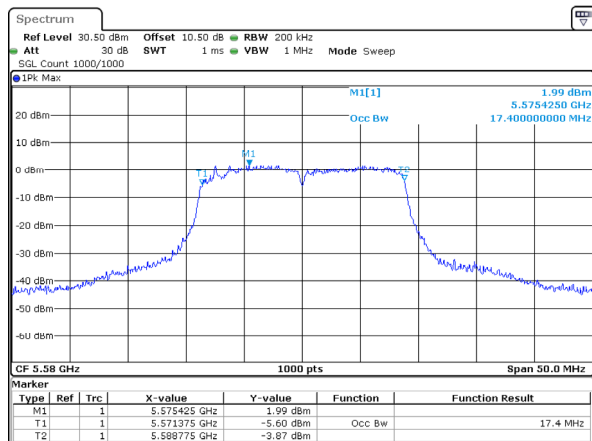
802.11ac20_5580MHz_Chain 0
