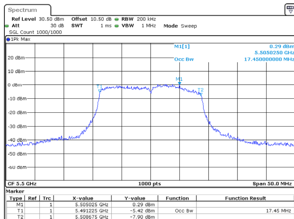
802.11ac20_5500MHz_Chain 2
