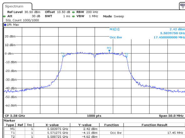
802.11ac20_5580MHz_Chain 2
