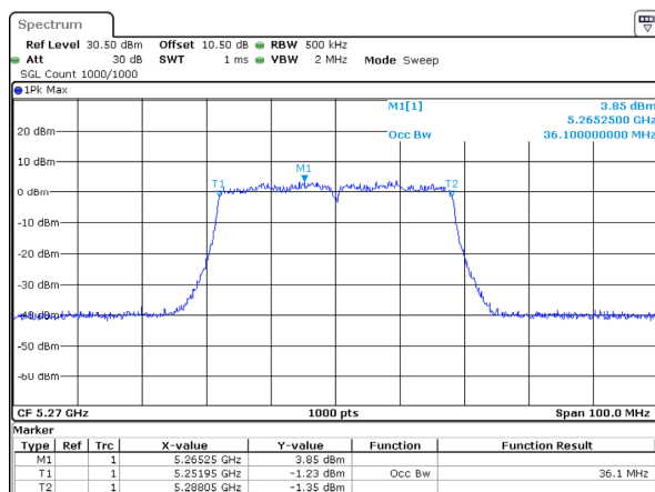
802.11ac40_5270MHz_Chain 3
