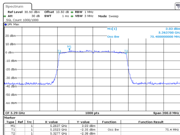
802.11ac80_5290MHz_Chain 1
