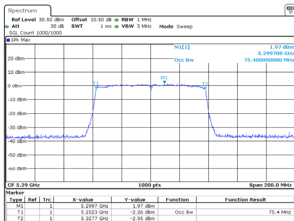
802.11ac80_5290MHz_Chain 0
