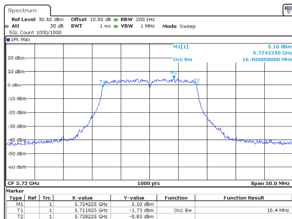
802.11a_5720MHz_Chain 2
