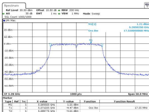
802.11ac20_5280MHz_Chain 0
