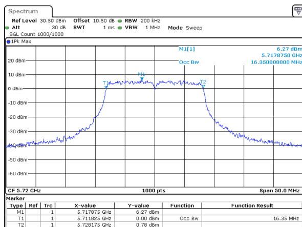
802.11a_5720MHz_Chain 1
