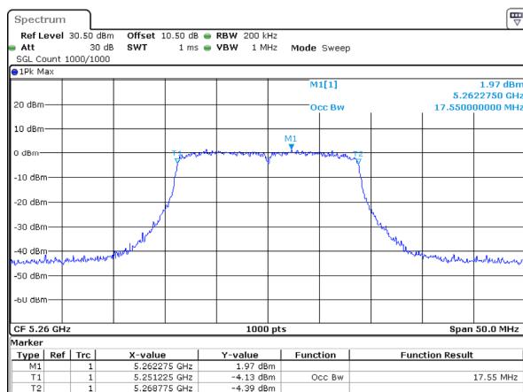
802.11ac20_5260MHz_Chain 0
