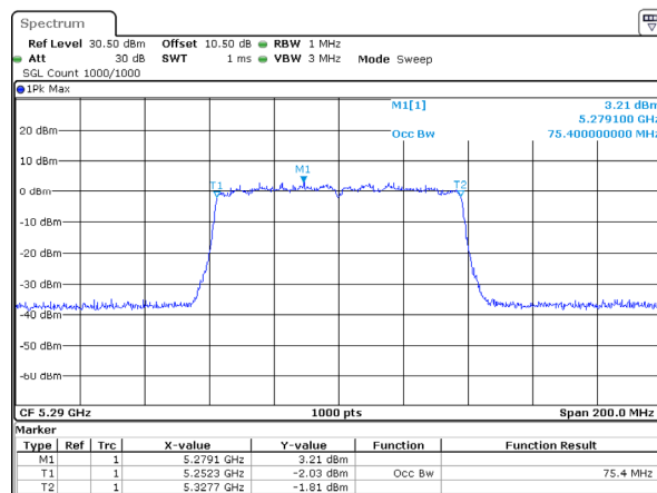
802.11ac80_5290MHz_Chain 3
