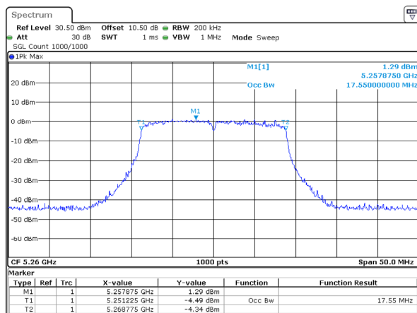
802.11ac20_5260MHz_Chain 1
