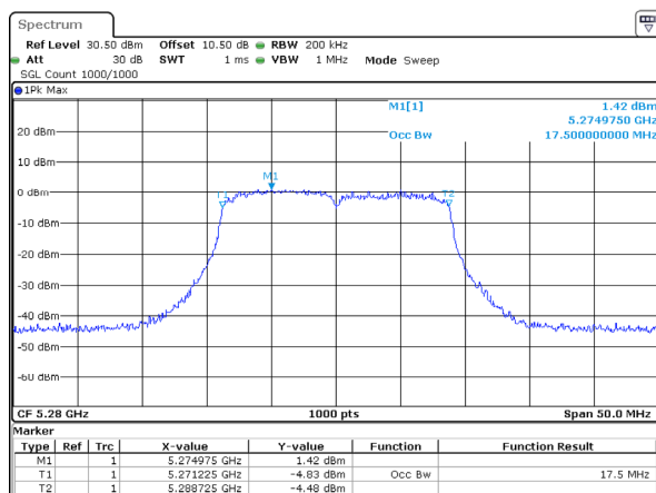
802.11ac20_5280MHz_Chain 2
