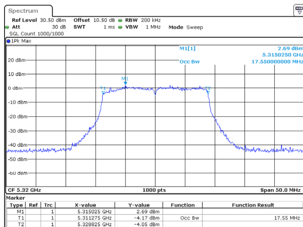
802.11ac20_5320MHz_Chain 3
