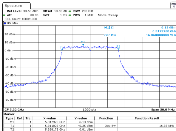
802.11a_5320MHz_Chain 3
