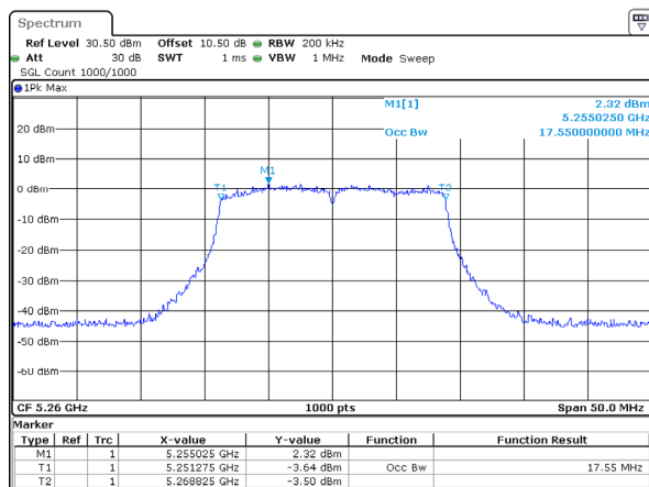
802.11ac20_5260MHz_Chain 3
