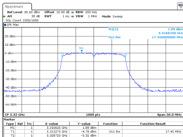
802.11ac20_5320MHz_Chain 2
