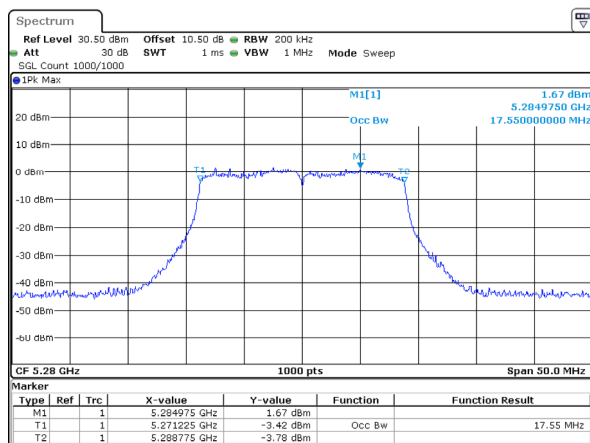
802.11ac20_5280MHz_Chain 3
