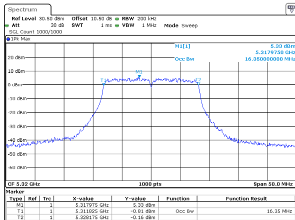
802.11a_5320MHz_Chain 2
