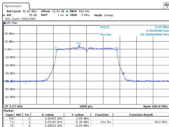
802.11ac40_5270MHz_Chain 1
