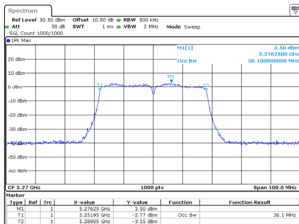
802.11ac40_5270MHz_Chain 2
