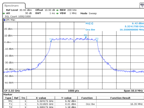
802.11a_5320MHz_Chain 1
