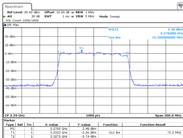
802.11ac80_5290MHz_Chain 2
