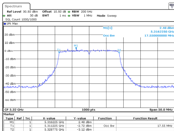
802.11ac20_5320MHz_Chain 1
