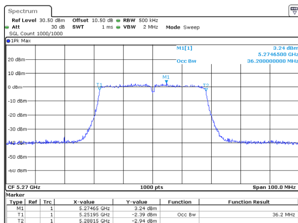
802.11ac40_5270MHz_Chain 0
