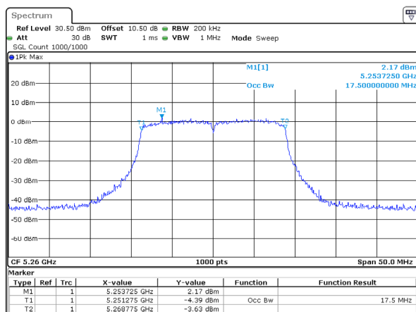
802.11ac20_5260MHz_Chain 2
