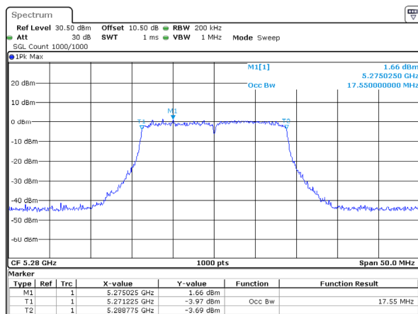
802.11ac20_5280MHz_Chain 1
