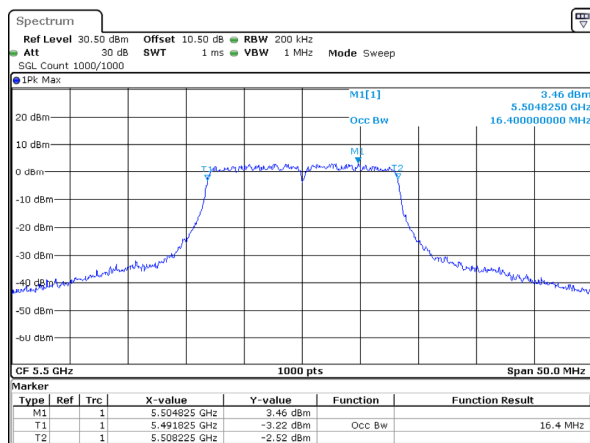
802.11a_5500MHz_Chain 2
