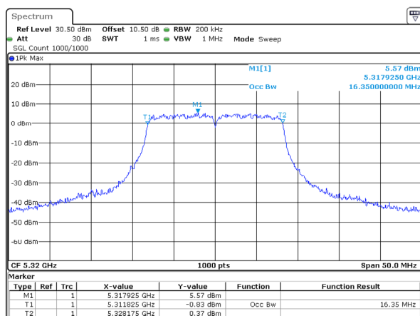
802.11a_5320MHz_Chain 0
