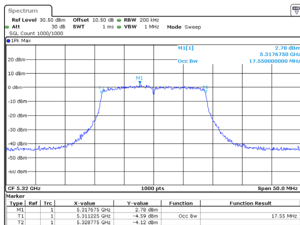
802.11ac20_5320MHz_Chain 0
