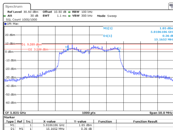
802.11ac20_5825MHz_Chain 3
