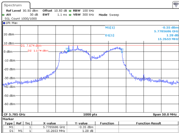
802.11ac20_5785MHz_Chain 2
