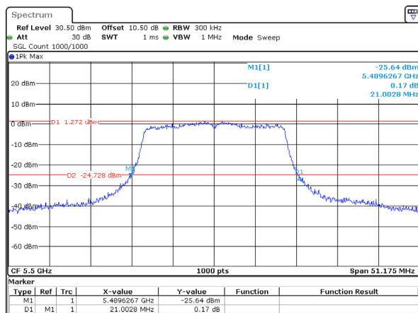
802.11ac20_5500MHz_Chain 0
