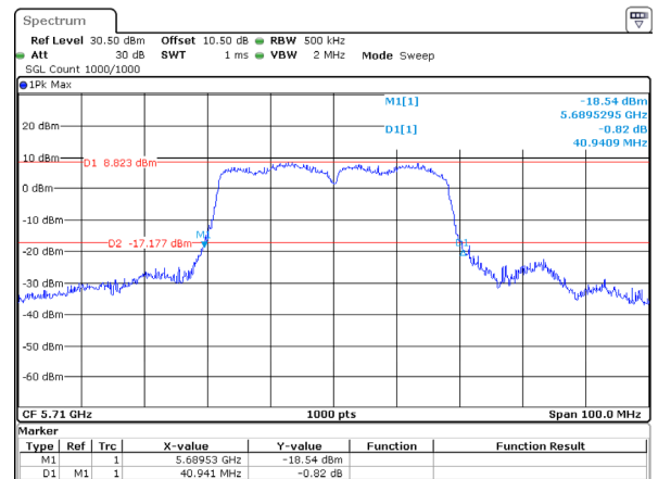
802.11ac40_5710MHz_Chain 0
