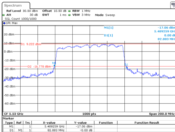
802.11ac80_5530MHz_Chain 0
