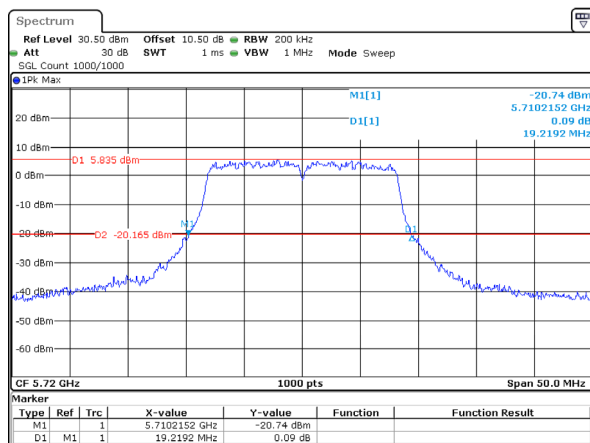
802.11a_5720MHz_Chain 3
