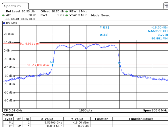
802.11ac80_5610MHz_Chain 1
