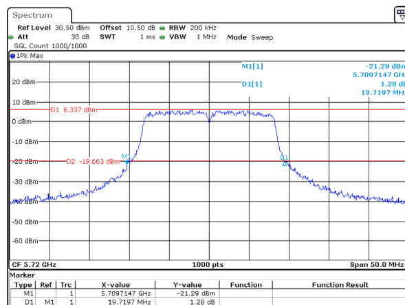
802.11a_5720MHz_Chain 1
