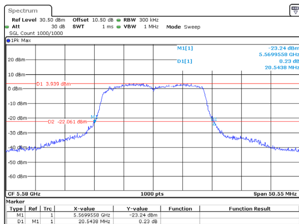
802.11ac20_5580MHz_Chain 0
