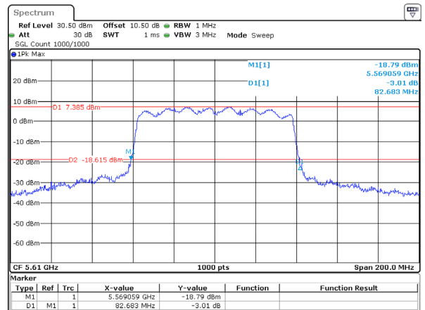
802.11ac80_5610MHz_Chain 0
