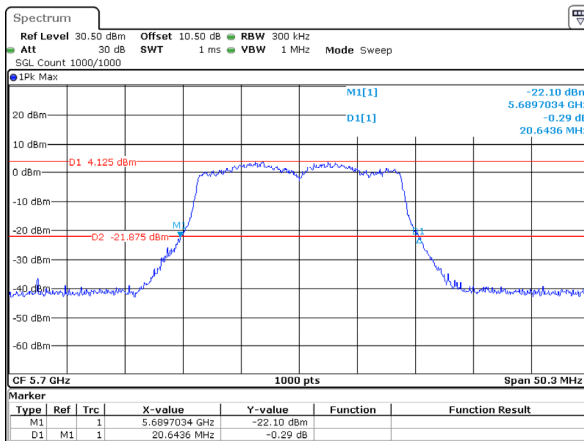
802.11ac20_5700MHz_Chain 3
