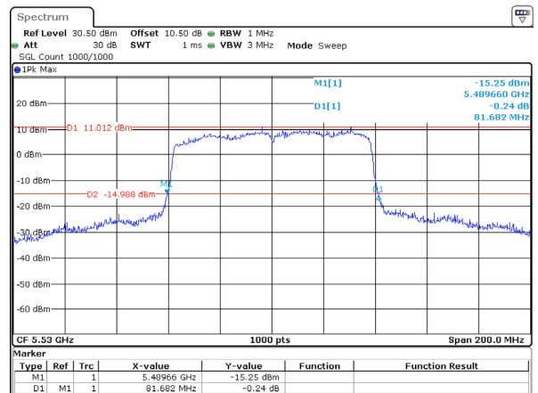
802.11ac80_5530MHz_Chain 1
