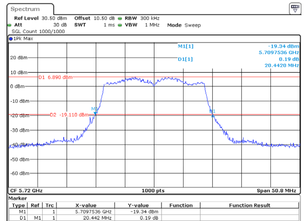
802.11ac20_5720MHz_Chain 3
