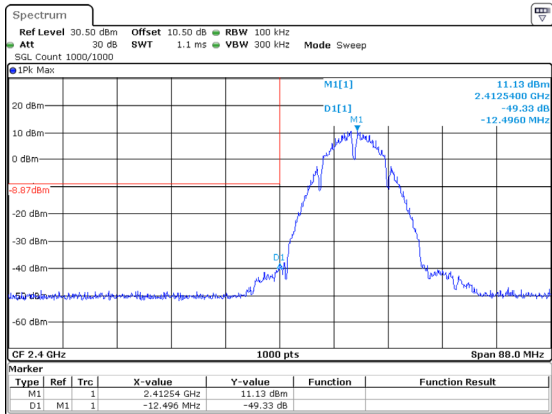
802.11b_2412MHz_Chain 3
