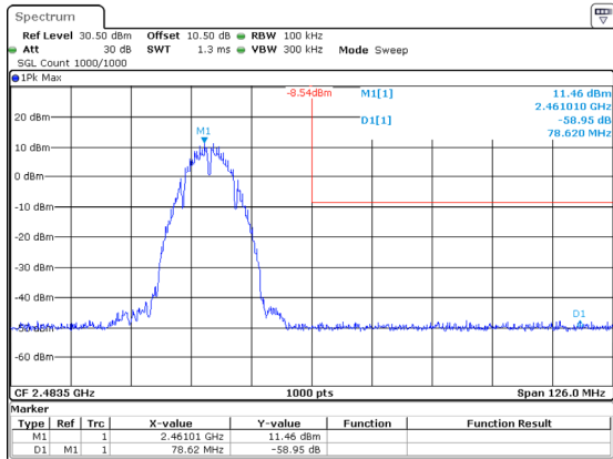
802.11b_2462MHz_Chain 3
