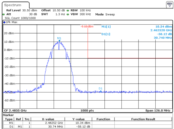
802.11b_2462MHz_Chain 2
