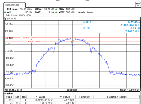
802.11b_2462MHz_Chain 3
