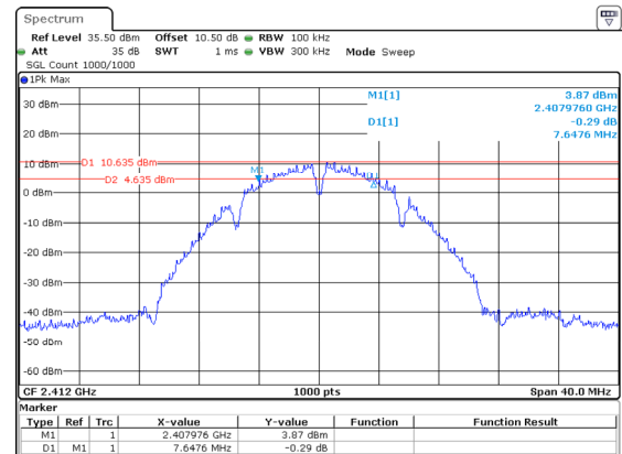
802.11b_2412MHz_Chain 3
