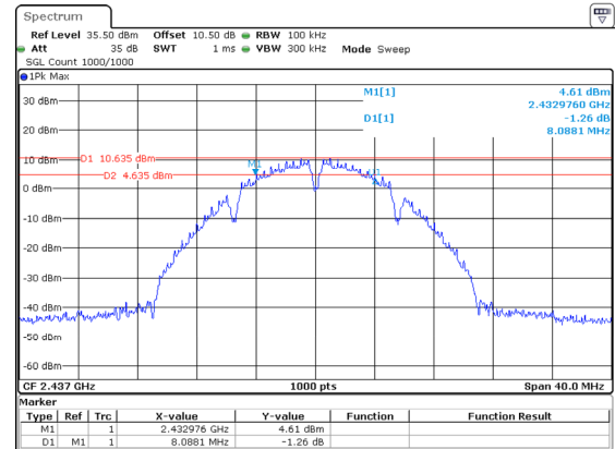
802.11b_2437MHz_Chain 2
