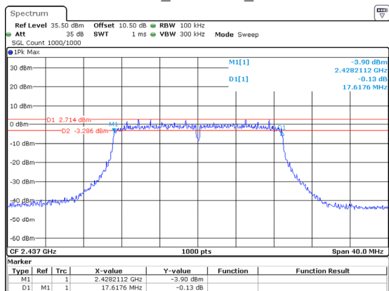
802.11n20_2437MHz_Chain 3
