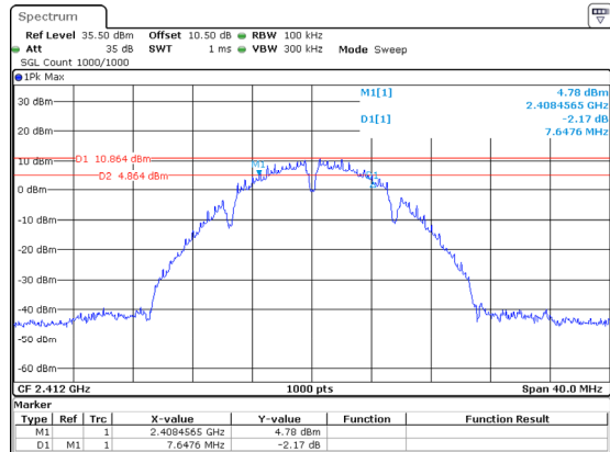
802.11b_2412MHz_Chain 2
