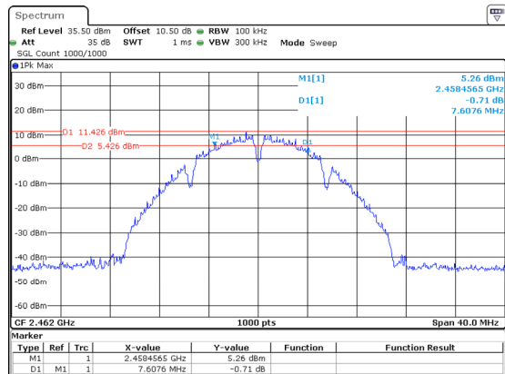
802.11b_2462MHz_Chain 2
