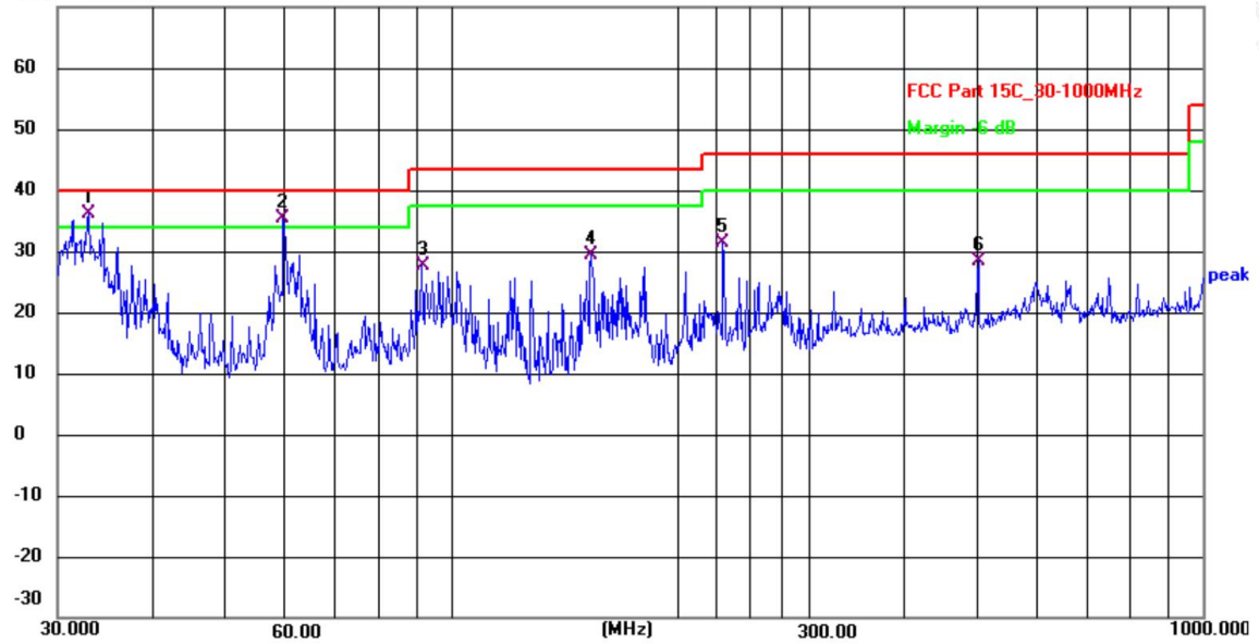
Horizontal 70.0 dBuV/m
