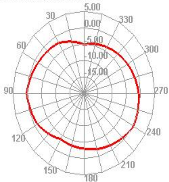
2450.000MHz H
