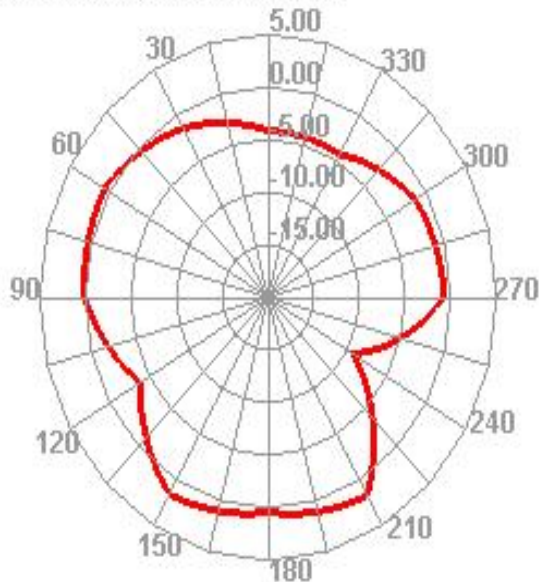
2450.000MHz E2
