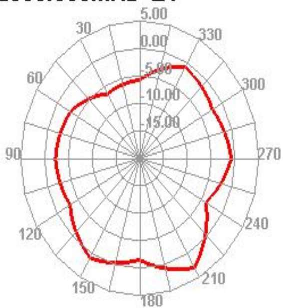
2500.000MHz E1
