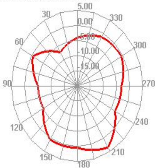
2450.000MHz E1
