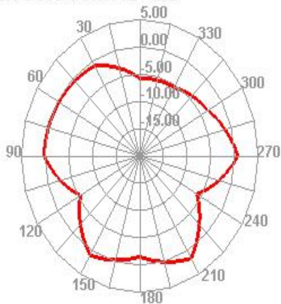
2500.000MHz E2
