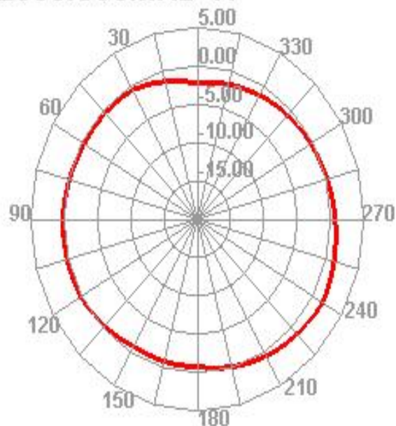
2500.000MHz H
