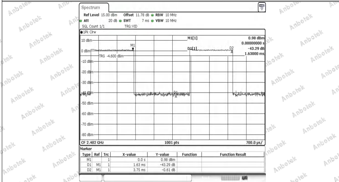
NTNV-2DH5-Ant1-2402
