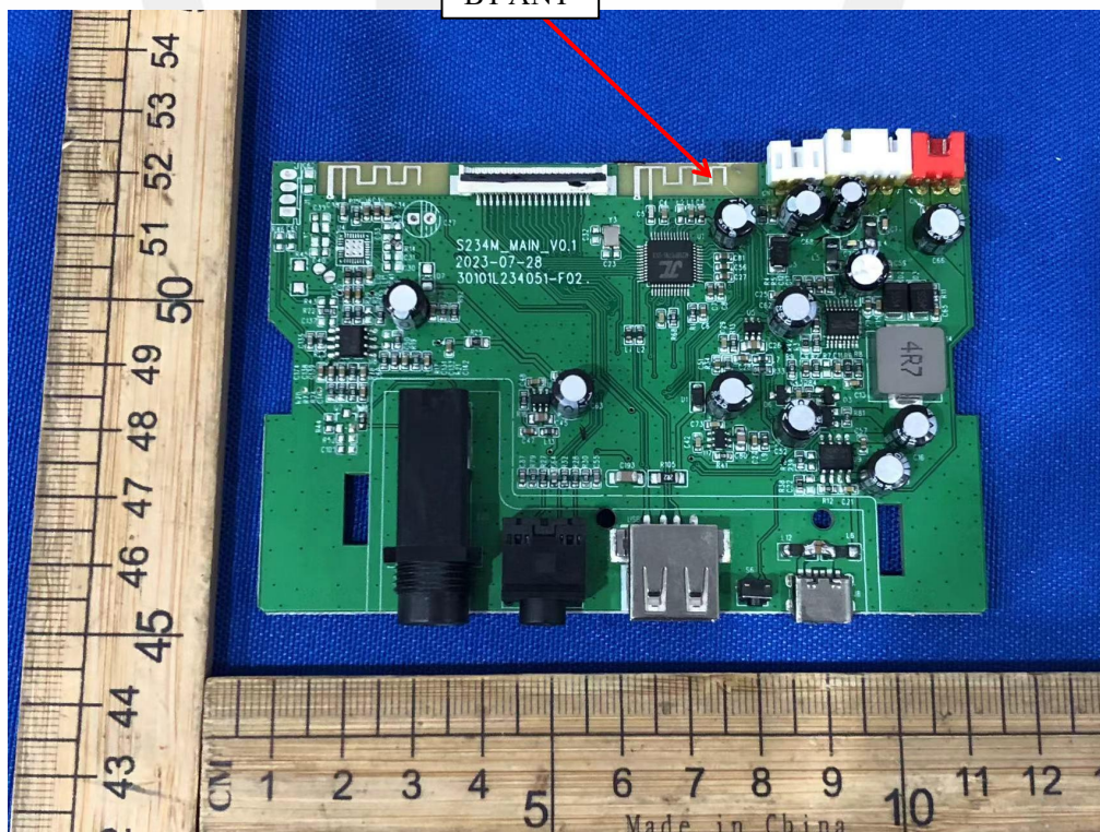
BT ANT
