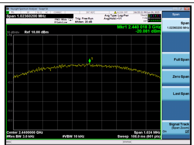
BLE 1Mbps 2440MHz
