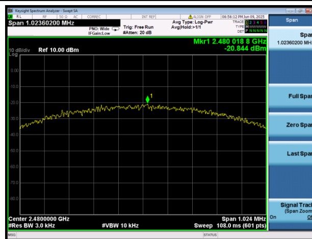
BLE 1Mbps 2480MHz
