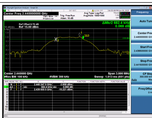
BLE 1Mbps 2440MHz
