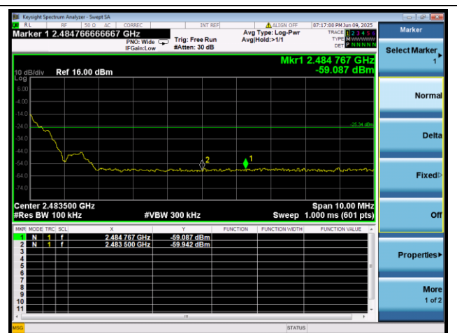
BLE 2Mbps 2478MHz
