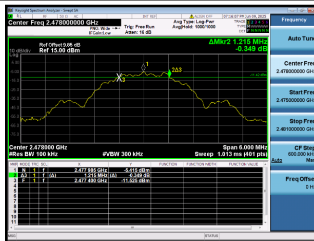
BLE 2Mbps 2478MHz
