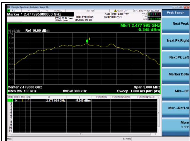
BLE 2Mbps 2478MHz
