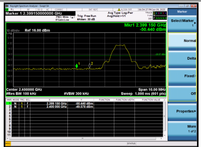
BLE 1Mbps 2402MHz
