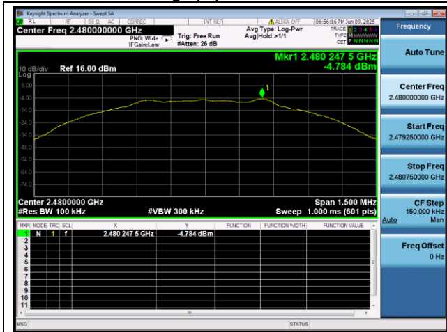
BLE 1Mbps 2480MHz
