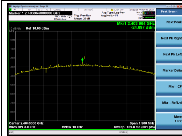
BLE 2Mbps 2404MHz
