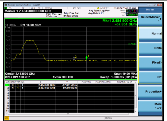
BLE 1Mbps 2480MHz
