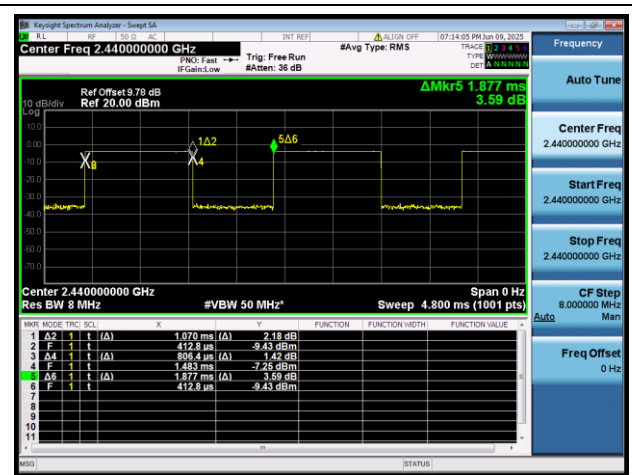
BLE 2Mbps 2440MHz
