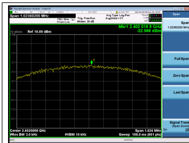
BLE 1Mbps 2402MHz
