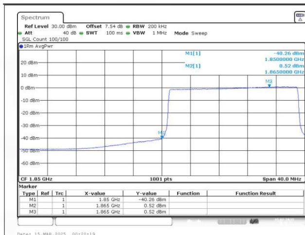
Band2 QPSK BW=20MHz Channel=18700 RB Size=100 Position=#0
