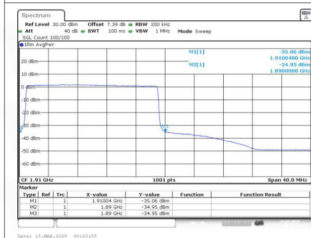
Band2 QPSK BW=20MHz Channel=19100 RB Size=100 Position=#0
