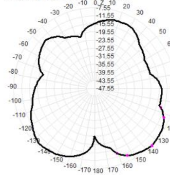
2500.0MHz Total(E2-YZ), Max=-7.55dBi
