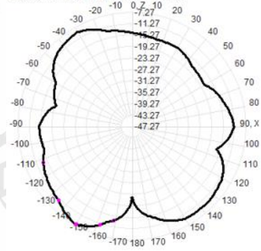
2480.0MHz Total(E1-XZ), Max=-7.94dBi
