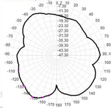
2470.0MHz Total(E1-XZ), Max=-7.76dBi
