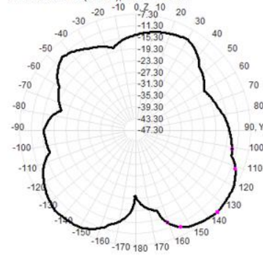
2470.0MHz Total(E2-YZ), Max=-7.27dBi
