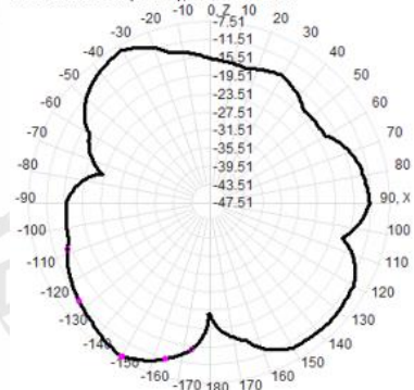
2440.0MHz Total(E1-XZ), Max=-8.52dBi
