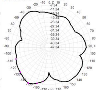
2450.0MHz Total(E1-XZ), Max=-7.99dBi
