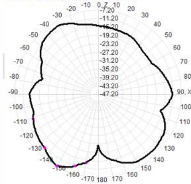
2490.0MHz Total(E1-XZ), Max=-8.46dBi
