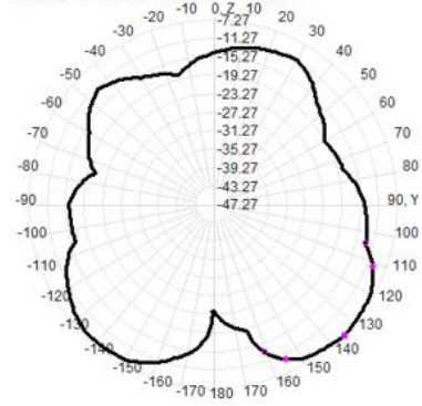
2480.0MHz Total(E2-YZ), Max=-7.20dBi
