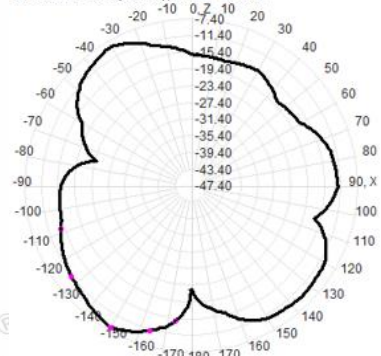
2430.0MHz Total(E1-XZ), Max=-8.48dBi
