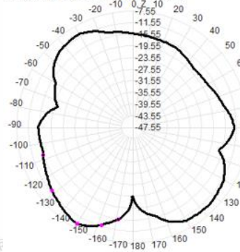
2500.0MHz Total(E1-XZ), Max=-9.31dBi
