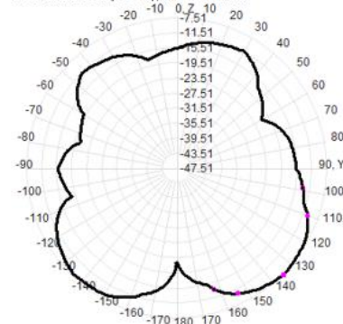
2440.0MHz Total(E2-YZ), Max=-7.52dBi
