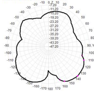
2490.0MHz Total(E2-YZ), Max=-7.18dBi
