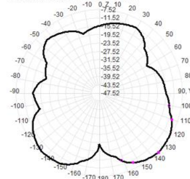
2450.0MHz Total(E2-YZ), Max=-7.34dBi
