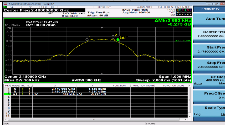
BLE 1M-Ant1-2480-PASS
