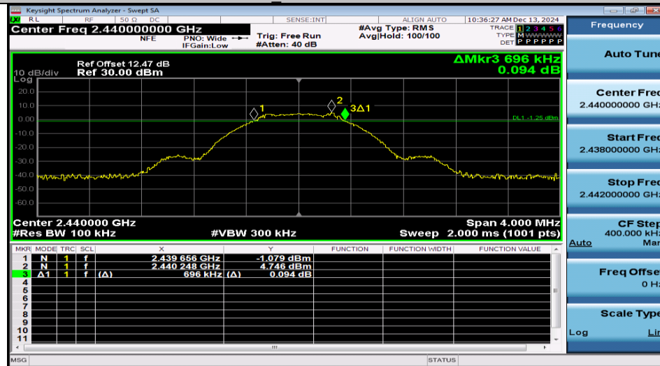
BLE 1M-Ant1-2440-PASS
