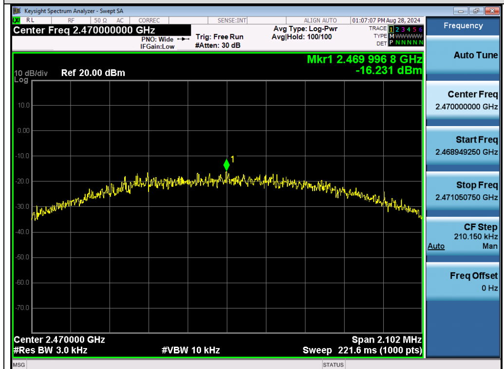
Test_Graph_GFSK_ANT1_2470_PSD
