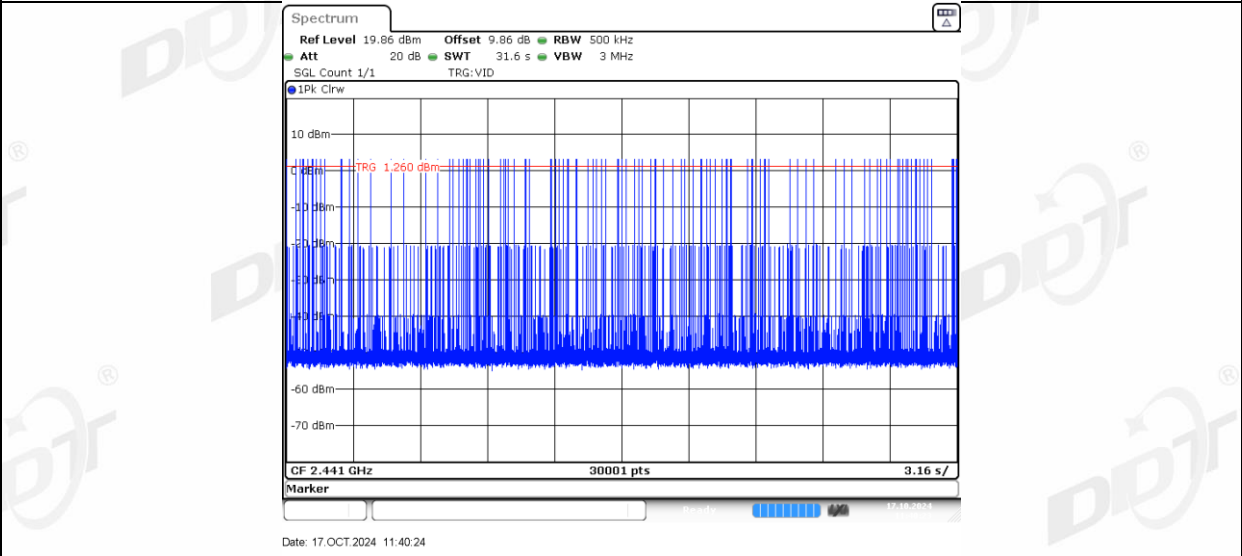
2DH1_Left side_Hop
