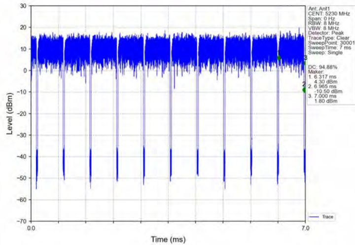
802.11n(HT40)_HCH_5230MHz_Ant1_NTNV
