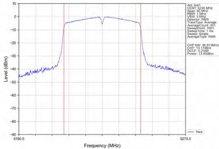
802.11n(HT40)_HCH_5230MHz_Ant1_NTNV
