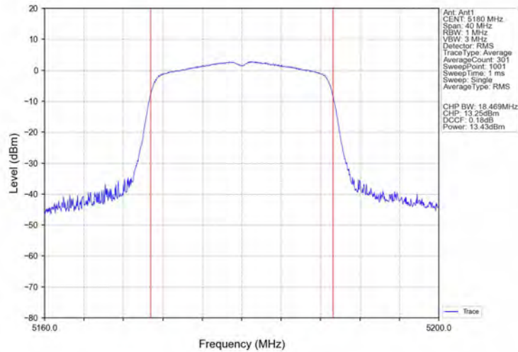
802.11n(HT20)_LCH_5180MHz_Ant1_NTNV
