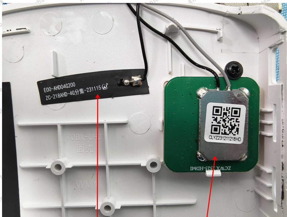
LTE DIV ANT
